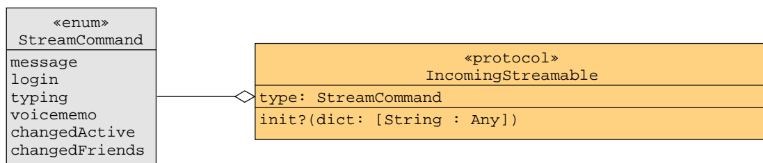
Abbildung 7.14: Klassendiagramm für das Protokoll IncomingStreamable
