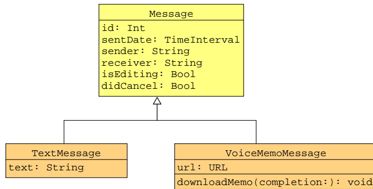
Abbildung 5.8: Klassendiagramm für die Model-Klasse einer Nachricht
