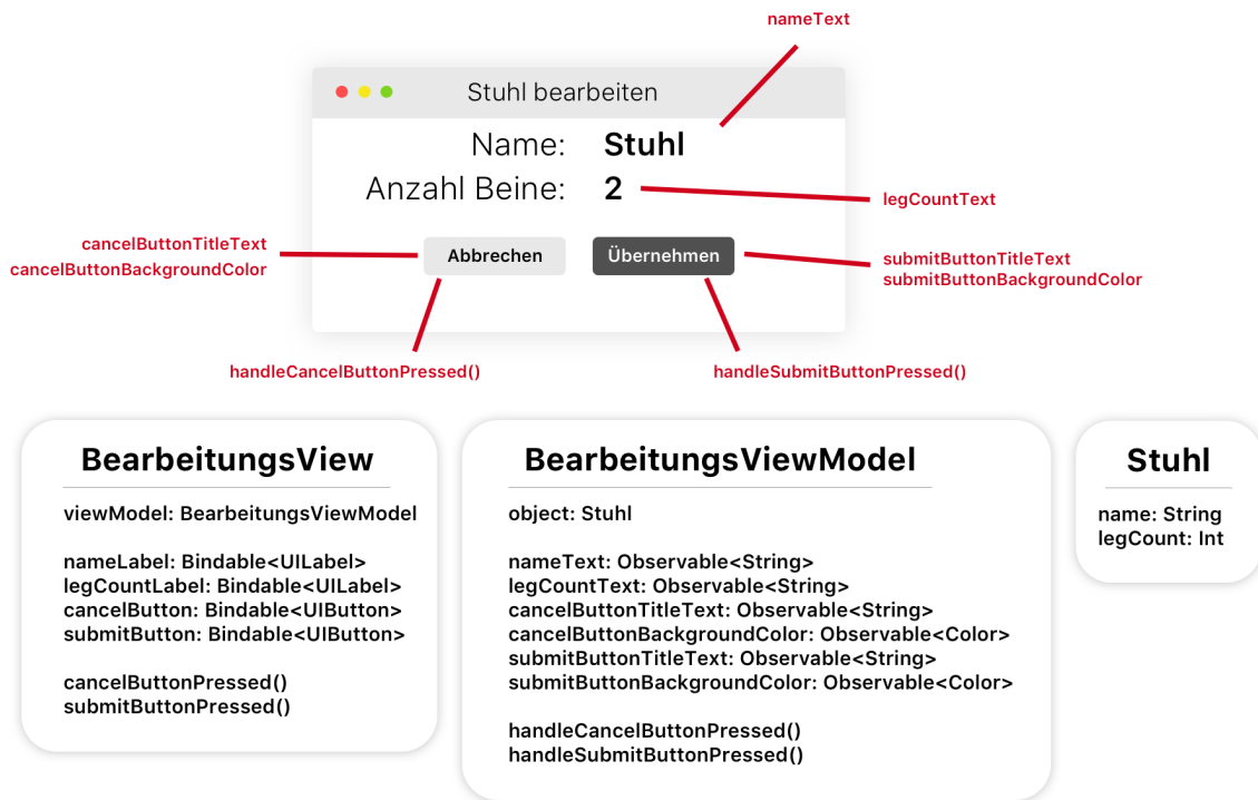
Abbildung 5.6: Visualisierung eines ViewModels für die BearbeitungsView
