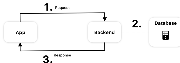
Abbildung 6.1: Visualisierung einer beispielhaften HTTP-Anfrage der App zum Backend
