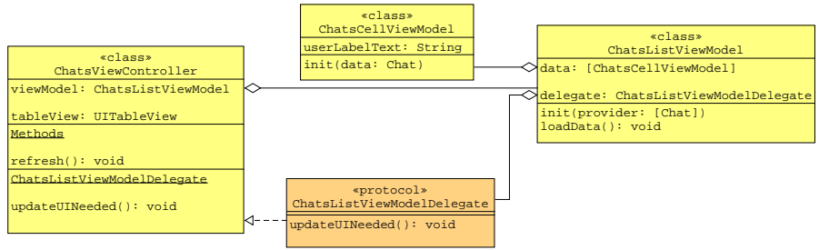
Abbildung 5.12: Klassendiagramm für einen Entwurf von ChatsViewController, ChatsListViewModel und ChatsCellViewModel
