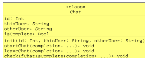
Abbildung 7.20: Klassendiagramm für den Aufbau des Chat-Modells
