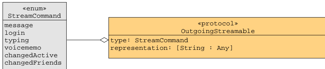
Abbildung 7.13: Klassendiagramm für das Protokoll OutgoingStreamable
