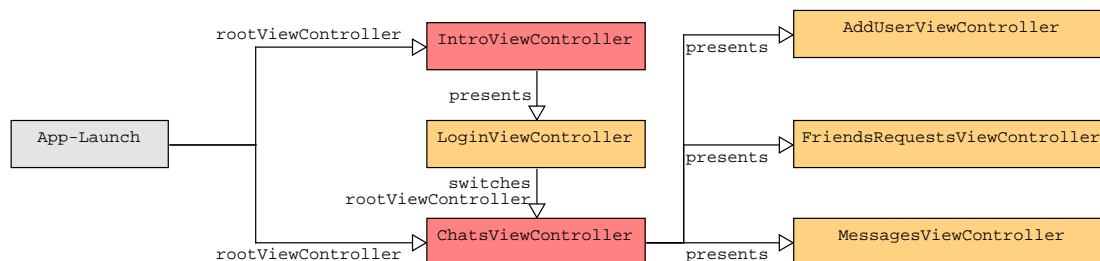
Abbildung 7.4: Hierarchie aller ViewController in M2
