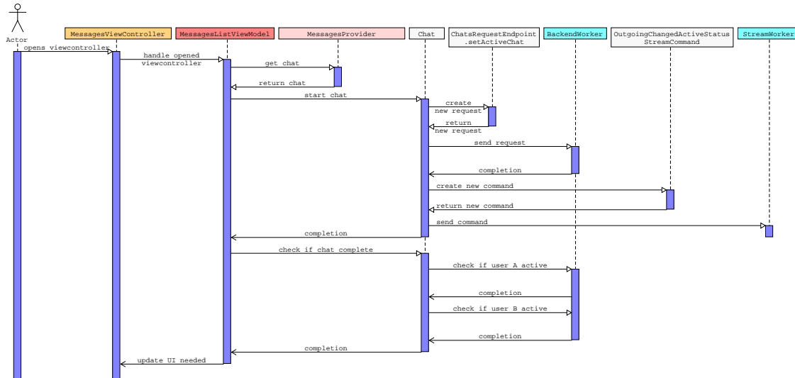
Abbildung 7.19: Sequenzdiagramm zum Ablauf des Chat-Startes
