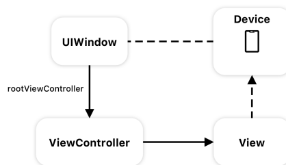
Abbildung 7.2: Hierarchie der Darstellung eines ViewControllers unter iOS
