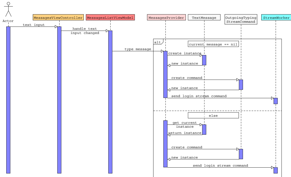
Abbildung 7.28: Sequenzdiagramm eines eingetippten Buchstabens einer Nachricht im MessagesViewController
