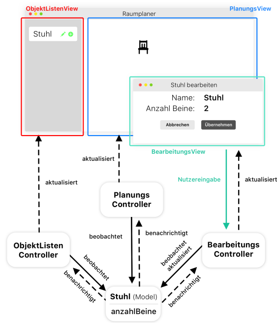
Abbildung 5.2: Visualisierung des Observer-Patterns
