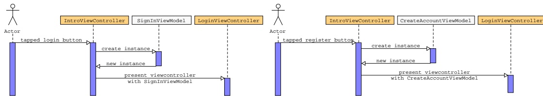
Abbildung 7.5: Sequenzdiagramm für Anmeldung (l) oder Registrierung (r) in M2
