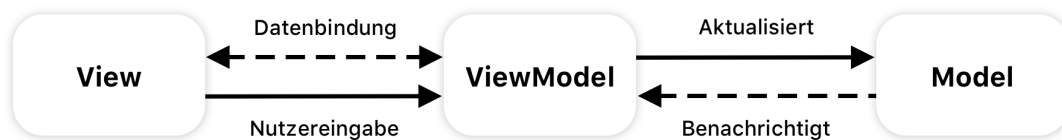
Abbildung 5.5: Visualisierung des MVVM Entwurfsmusters
