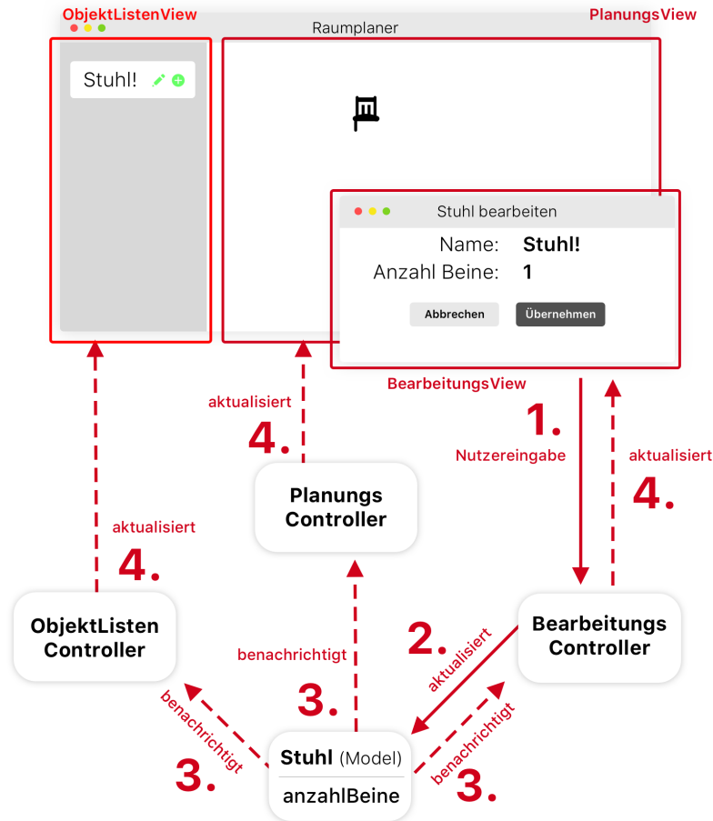
Abbildung 5.3: Ausgelöster Ablauf durch Nutzereingabe in BearbeitungsView mit Observer-Pattern
