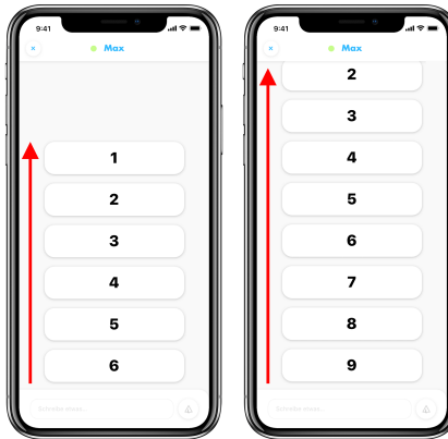
Abbildung 7.23: Bodenorientierte Anordnung der UITableView
