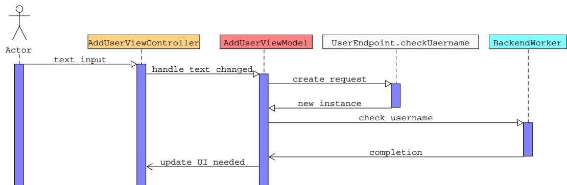
Abbildung 7.16: Sequenzdiagramm für eine Texteingabe im AddUserController
