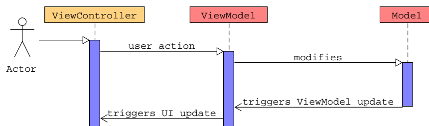
Abbildung 5.7: Sequenzdiagramm für die Nutzung des MVVM-Entwurfsmusters in M2
