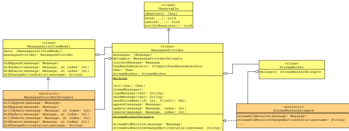
Abbildung 7.27: Klassendiagramm des MessagesProviders und seiner Abhängigkeiten
