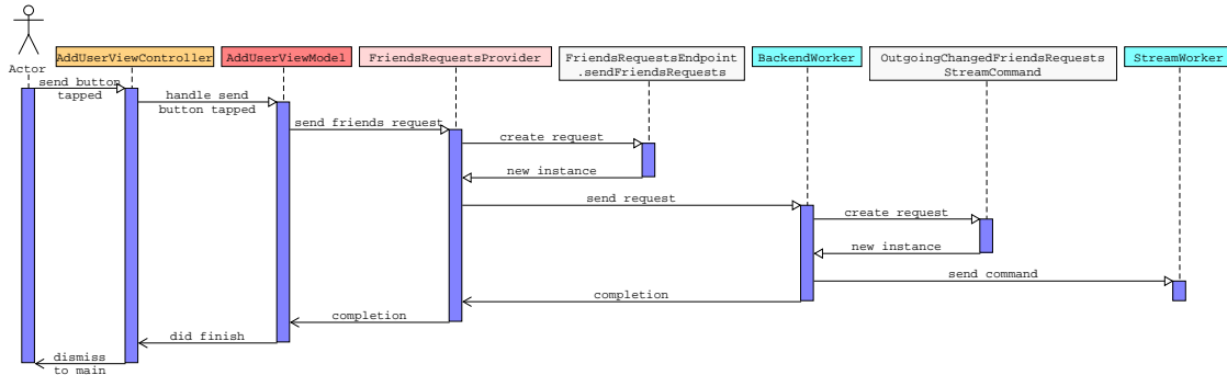
Abbildung 7.17: Sequenzdiagramm für das erfolgreiche Absenden einer Freundschaftsanfrage mit dem AddUserController
