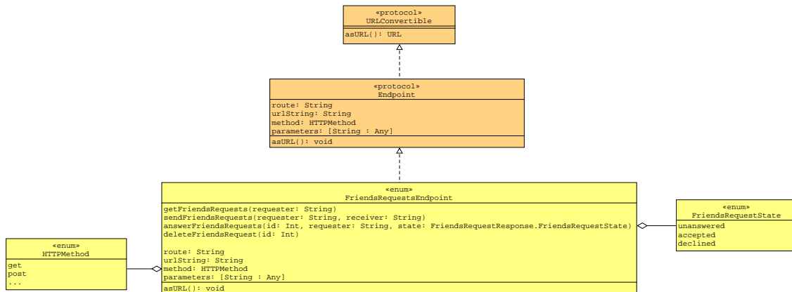
Abbildung 7.11: Klassendiagramm für die Implementierung des FriendsRequestsEndpoints
