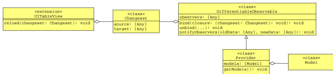
Abbildung 7.9: Klassendiagramm für die Implementierung von DifferenceKit in M2
