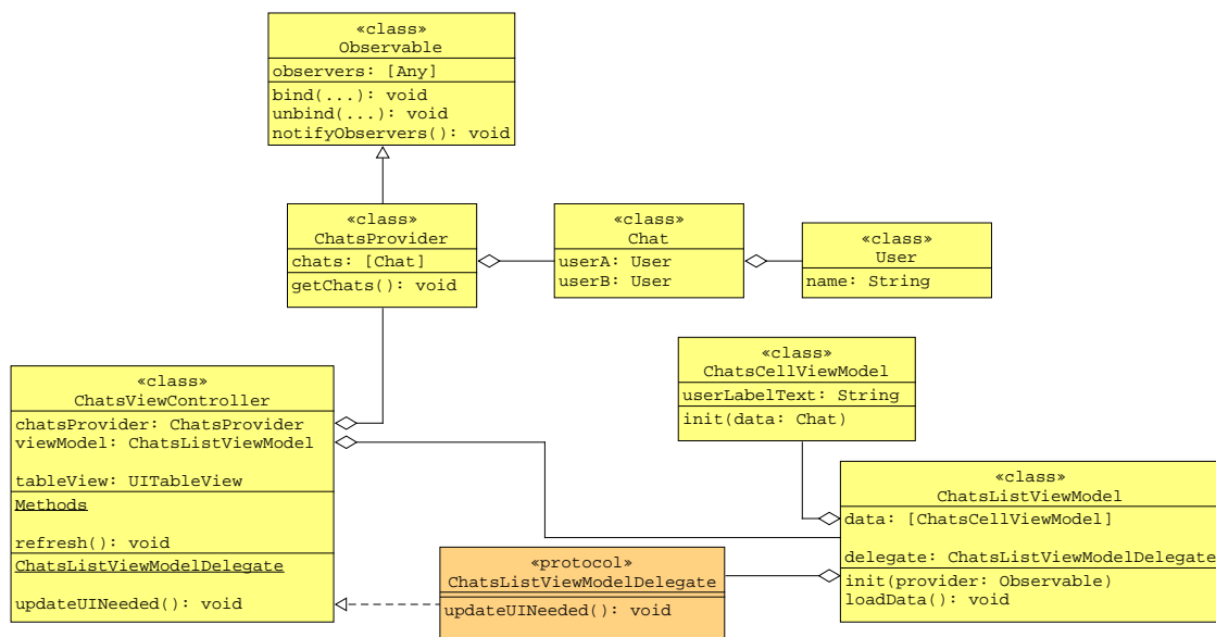
Abbildung 5.14: Klassendiagramm für einen Entwurf von ChatsViewController, ChatsListModel und ChatsCellViewModel inklusive ChatsProvider
