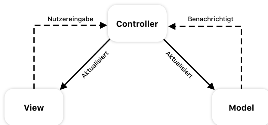
Abbildung 5.1: Visualisierung einer oftmals verwendeten Ausführung des Entwurfsmusters MVC (indirekte Assoziationen mit gestrichelten Pfeilen)
