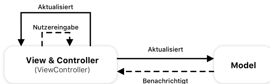
Abbildung 5.4: Visualisierung von MVC mit einem ViewController
