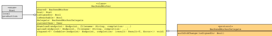
Abbildung 7.10: Klassendiagramm für die Implementierung des BackendWorkers
