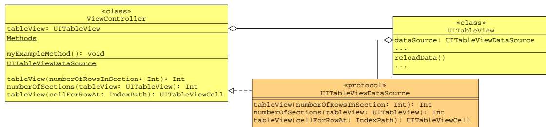
Abbildung 7.8: Beispielhaftes Klassendiagramm für die Implementierung einer UITableView inklusive UITableViewDataSource
