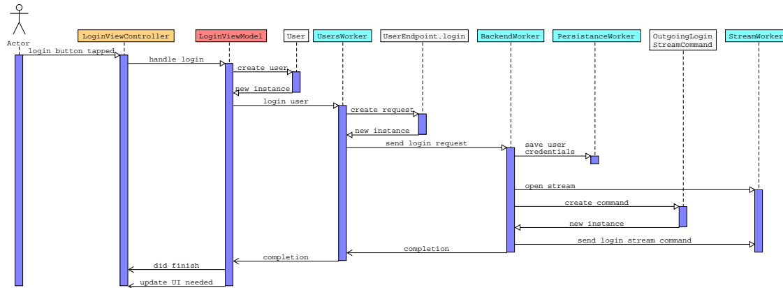
Abbildung 7.7: Sequenzdiagramm für die Anmeldung in M2
