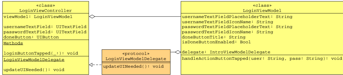
Abbildung 5.10: Klassendiagramm für einen Entwurf von LoginViewController und LoginViewModel
