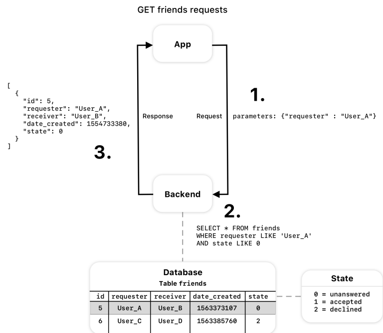
Abbildung 7.1: Visualisierung des gesamten Ablaufs einer HTTP-Anfrage von der App zum Backend
