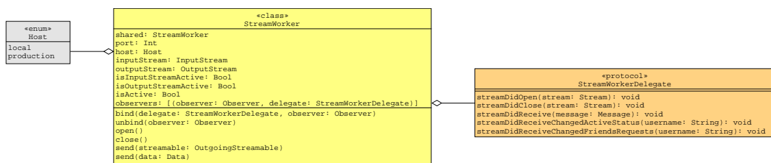
Abbildung 7.12: Klassendiagramm des StreamWorkers
