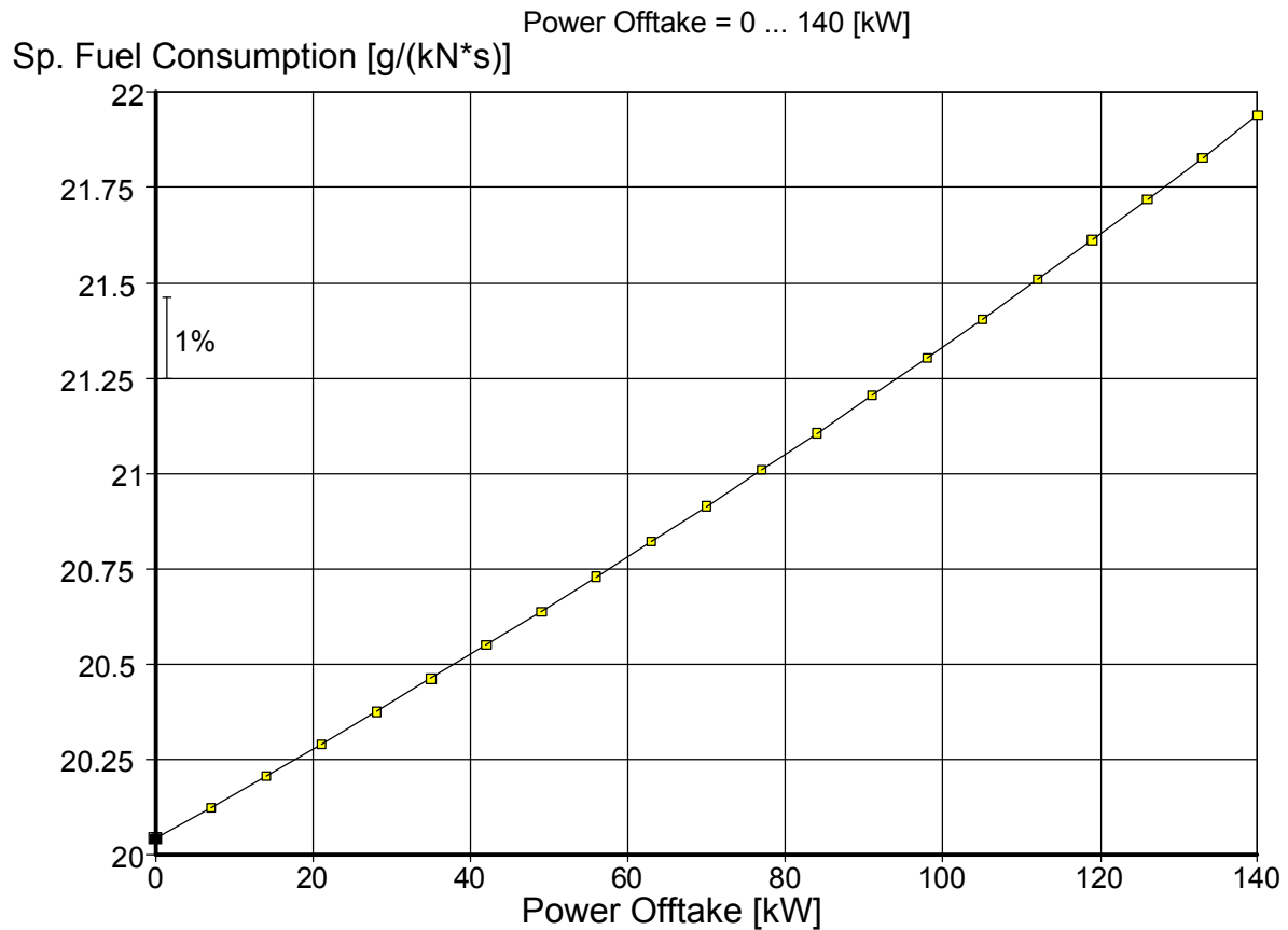
Bild 6.4 SFC über Wellenleistungsentnahme beim DWTT mit Integral Schubdüse
