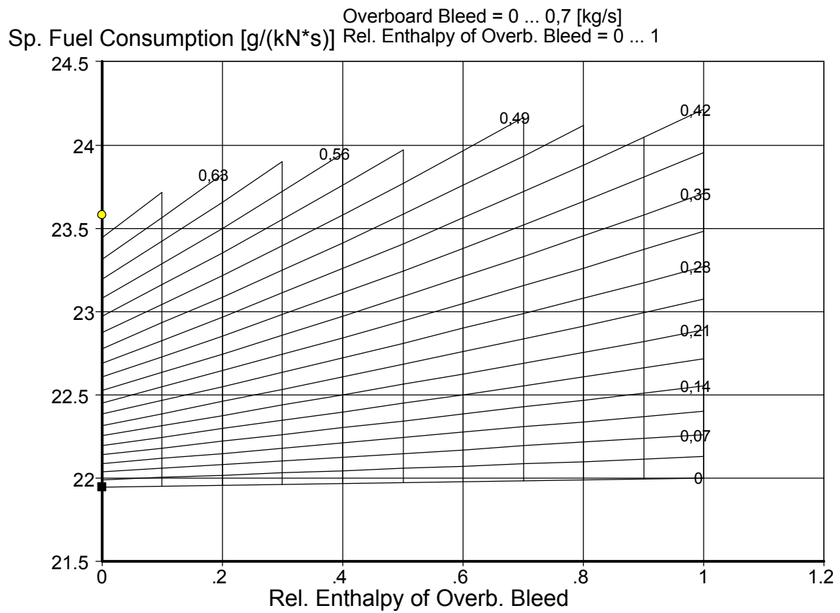
Bild 5.4 SFC über relativer Enthalpie beim ZWTT mit Integral Schubdüse
