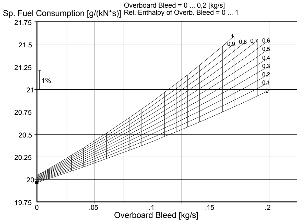
Bild 5.7 SFC über Zapfluftmassenstrom beim DWTT mit Integral Schubdüse
