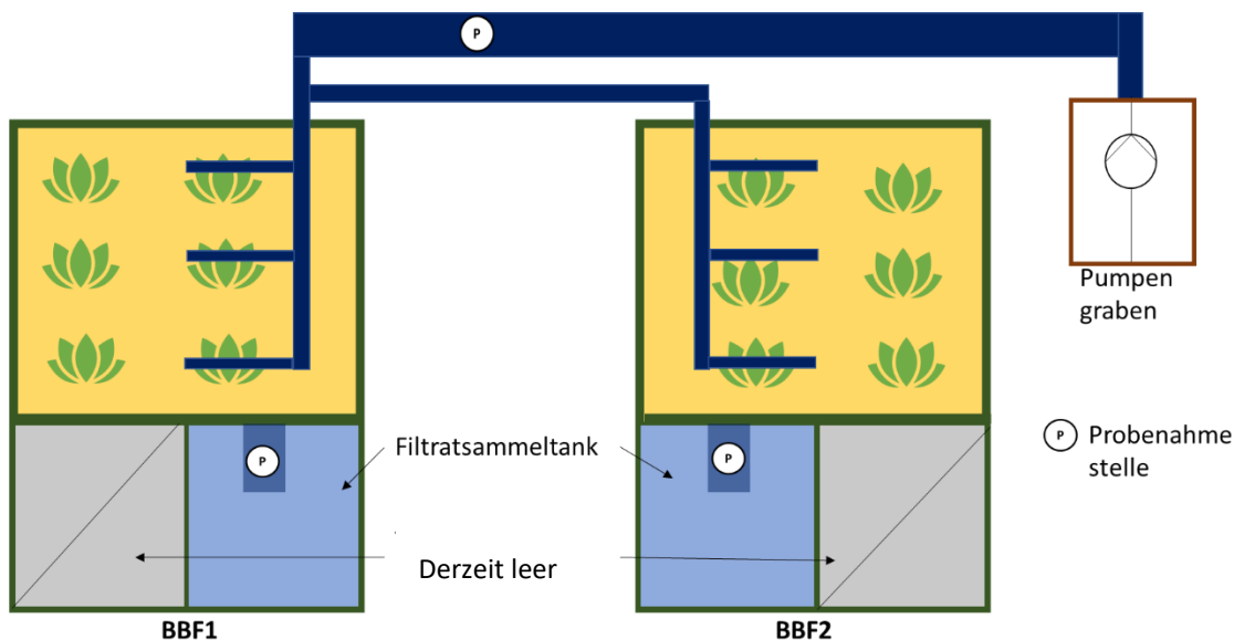
Abbildung 13: BBF1 und BBF2 mit Messstellen
