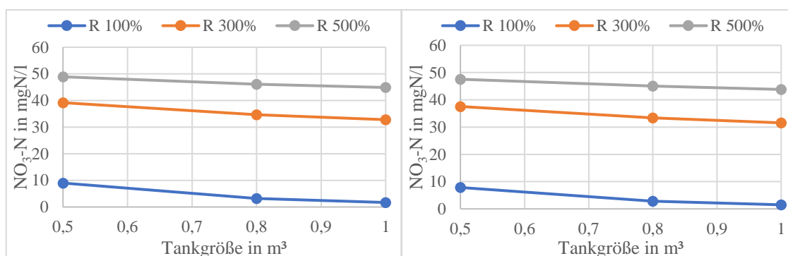
Abbildung 19: Links: \text{NO}_3\text{-N} Konzentration in mg/l aufgetragen über das Tankvolumen 0,5 m 3 , 0,8 m 3 und 1 m 3 für die Rezirkulationsraten von 100%, 300% und 500% (DT-CSTR). Rechts: \text{NO}_3\text{-N} Konzentration in mg/l aufgetragen über das Tankvolumen 0,5 m 3 , 0,8 m 3 und 1 m 3 für die Rezirkulationsraten von 100%, 300% und 500% (DT-MBBR).
