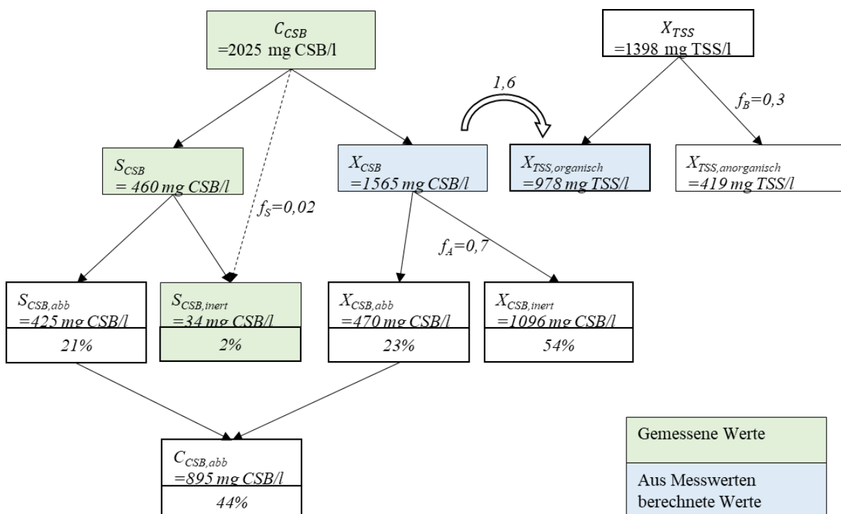
Abbildung 17: Verwendete CSB Fraktionierung für die Simulation
