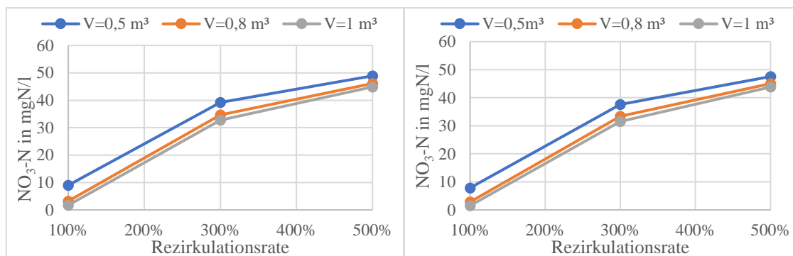
Abbildung 20: Links: \text{NO}_3\text{-N} Konzentration im Ablauf in mg/l aufgetragen über Filtrat Zuflüsse von 100%, 300% und 500% für die Tankvolumen 0,5 m 3 , 0,8 m 3 und 1 m 3 (DT-CSTR). Rechts: \text{NO}_3\text{-N} Konzentration im Ablauf in mg/l aufgetragen über Filtrat Zuflüsse von 100%, 300% und 500% für die Tankvolumen 0,5 m 3 , 0,8 m 3 und 1 m 3 (DT-MBBR).
