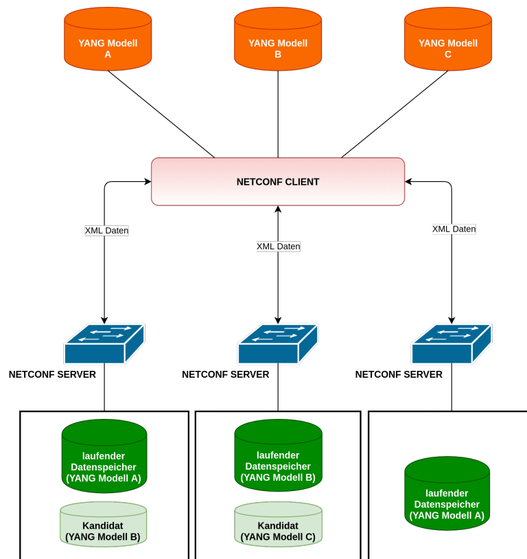
Abbildung 2.4: Server und Client in NETCONF
