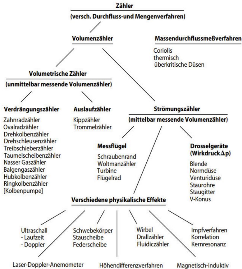
Abbildung 1: Übersicht verschiedener Durchfluss- und Mengemessverfahren [52, S. 794]
