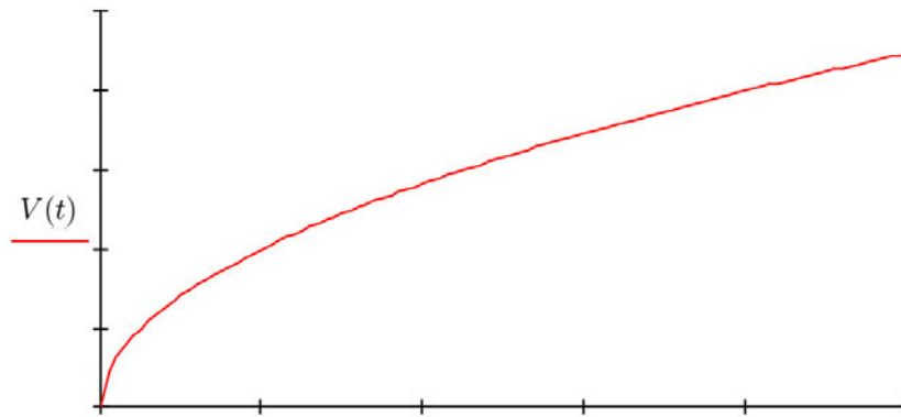
Abbildung 6: Filterkurve bei isobarer Betriebsweise [11, S. 8]
