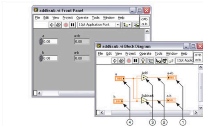
Abbildung 19: Beispiel für ein Blockdiagramm und das zugehörige Frontpanel [18]
