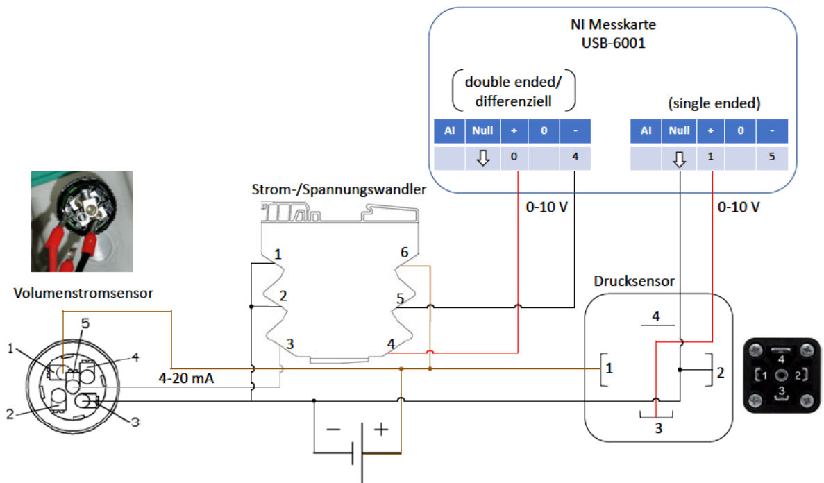
Abbildung 64: Elektrotechnische Verschaltung der Komponenten der Wirbelschichtversuchsanlage
