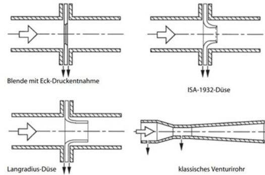
(b) Wirkdruckdrosselgeräte Übersicht nach DIN
