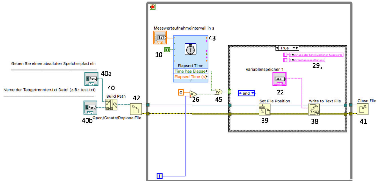
Abbildung 44: Datalogger
