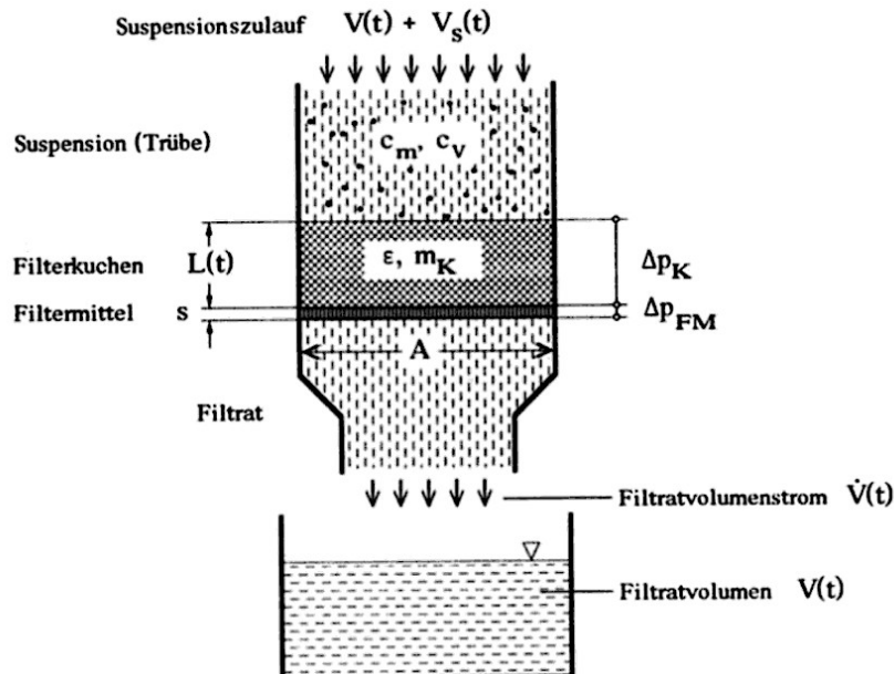
Abbildung 5: Filterkuchenmodell zur Ableitung der Filtergleichung, gemäß [42, S.100 ff.]
