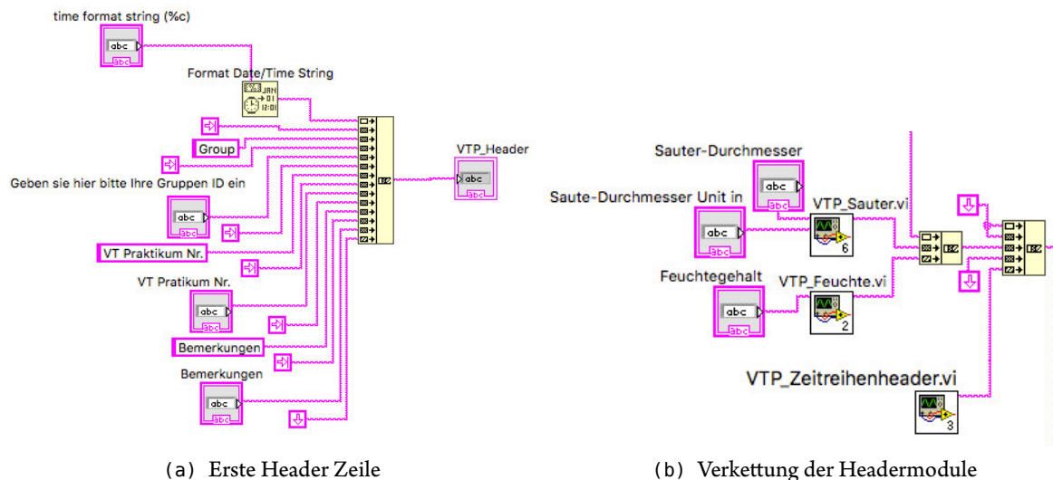
Abbildung 46: Modulare Header Sub VI's
