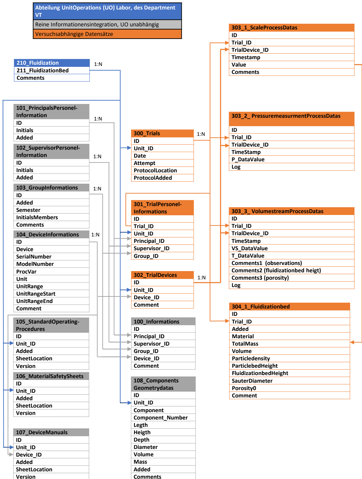
Abbildung 32: Datenstrukturentwurf einer relationalen Datenbank zur Beschreibung der Wirbelschicht Unit Operation, angelehnt an ISA-S95 und B2MML
