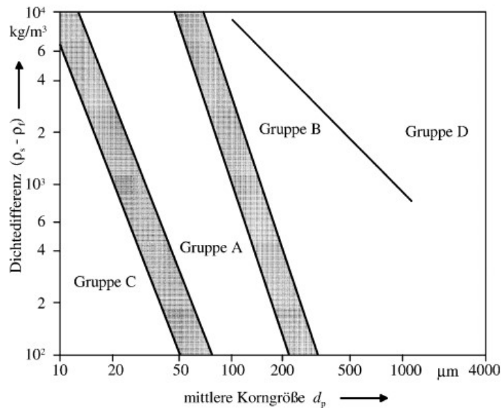
Abbildung 8: Klassifizierung von Schüttgütern nach Geldart [41, S. 1566 ff.]
