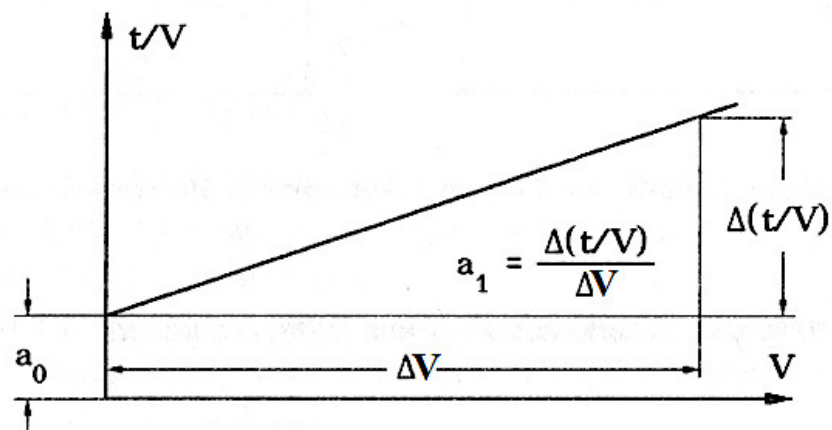
Abbildung 7: Filtergerade für die isobare Betriebsweise [42, S.102 ff.]
