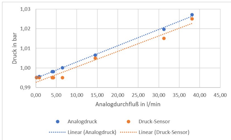
Abbildung 49: Analog-, Digitaldruckmessung als Funktion der analogen Volumenstrommesswerte
