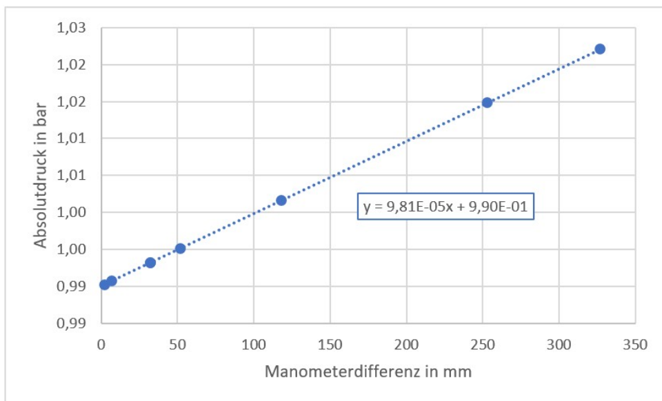
Abbildung 86: Manometerkennlinie; Druckdifferenz zzgl. 0,99 bar, laut digitalem Drucksensor am 17.12.20, um 13:02 Uhr
