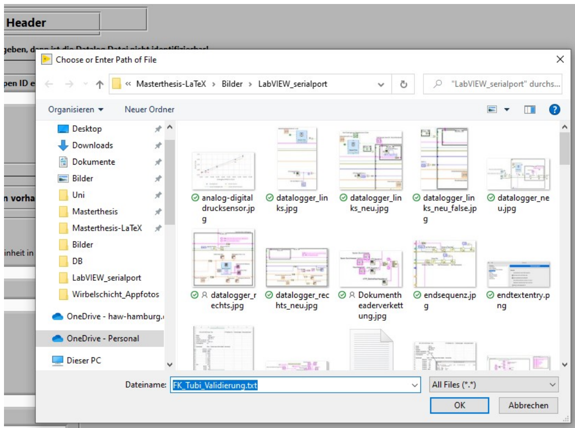
Abbildung 82: Dateialog
