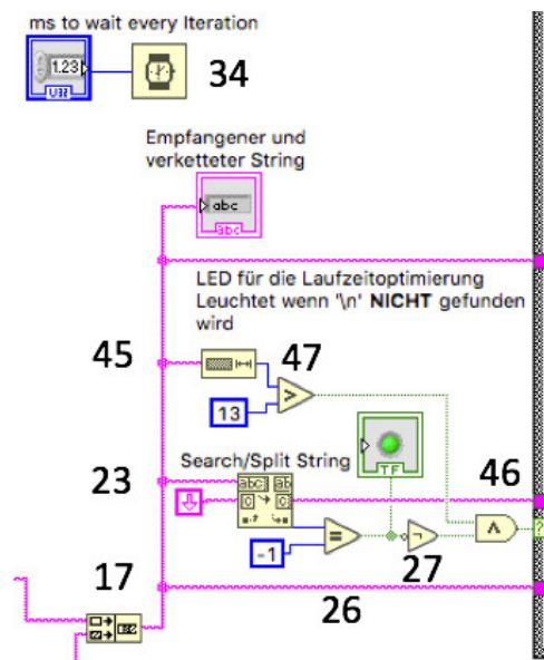
Abbildung 40: Slicing Bedingung
