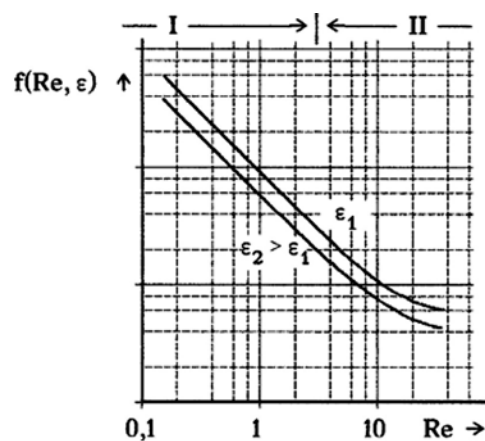
Abbildung 4: Widerstandsfunktion für die Durchströmung von Schüttgütern, gemäß [43, S. 146]
