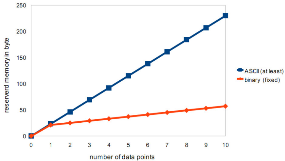
Abbildung 70: Speicherbedarfsvergleich ASCII/binär [15, S. 44]
