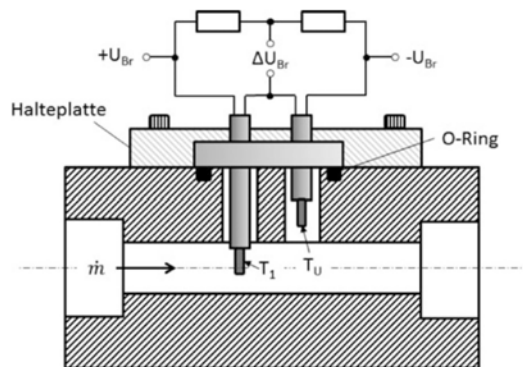
Abbildung 3: Prinzip eines thermischen Massendurchflusssensors [50, S. 656]
