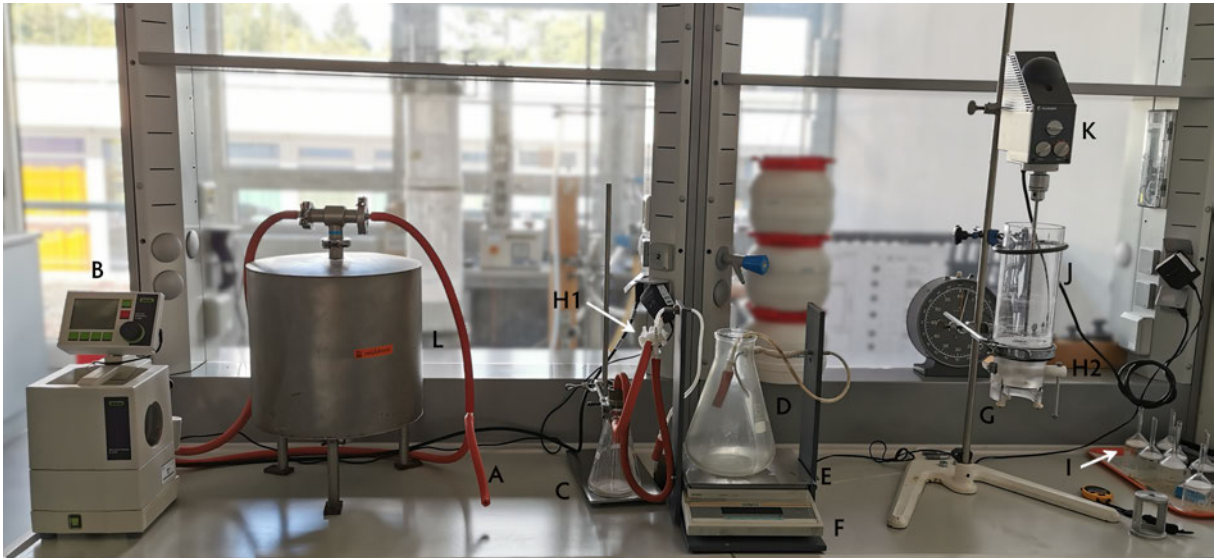
(a) Filterkuchenversuchsstand vor den Modifikationen
