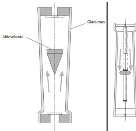
(a) Schwebekörperdurchflussmesser (links) Federscheibendurchflussmesser (rechts)
