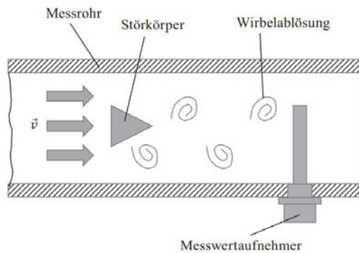
(e) Vortexsensor
