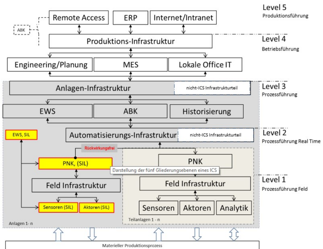
Abbildung 68: Hierarchische Gliederung eines ICS, gemäß ICS-Kompodium des Bundesamtes für Sicherheit in der Informationstechnik [40, S. 18]
