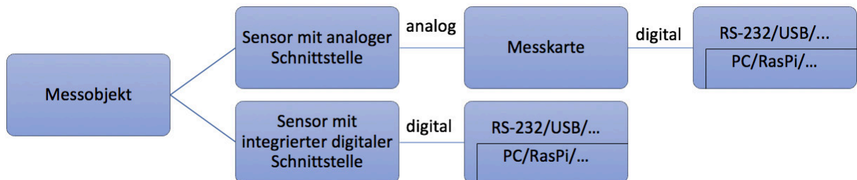
Abbildung 14: Anschluss eines Messgerätes an den PC, angelehnt an [7, S. 479]) oben mit Messkarte, unten mit digitaler Schnittstelle
