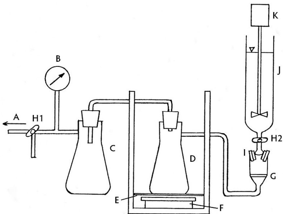
(b) Fließschema in Form einer schematischen Skizze der Filterkuchenversuchsanlage vor den Modifikationen [11]
