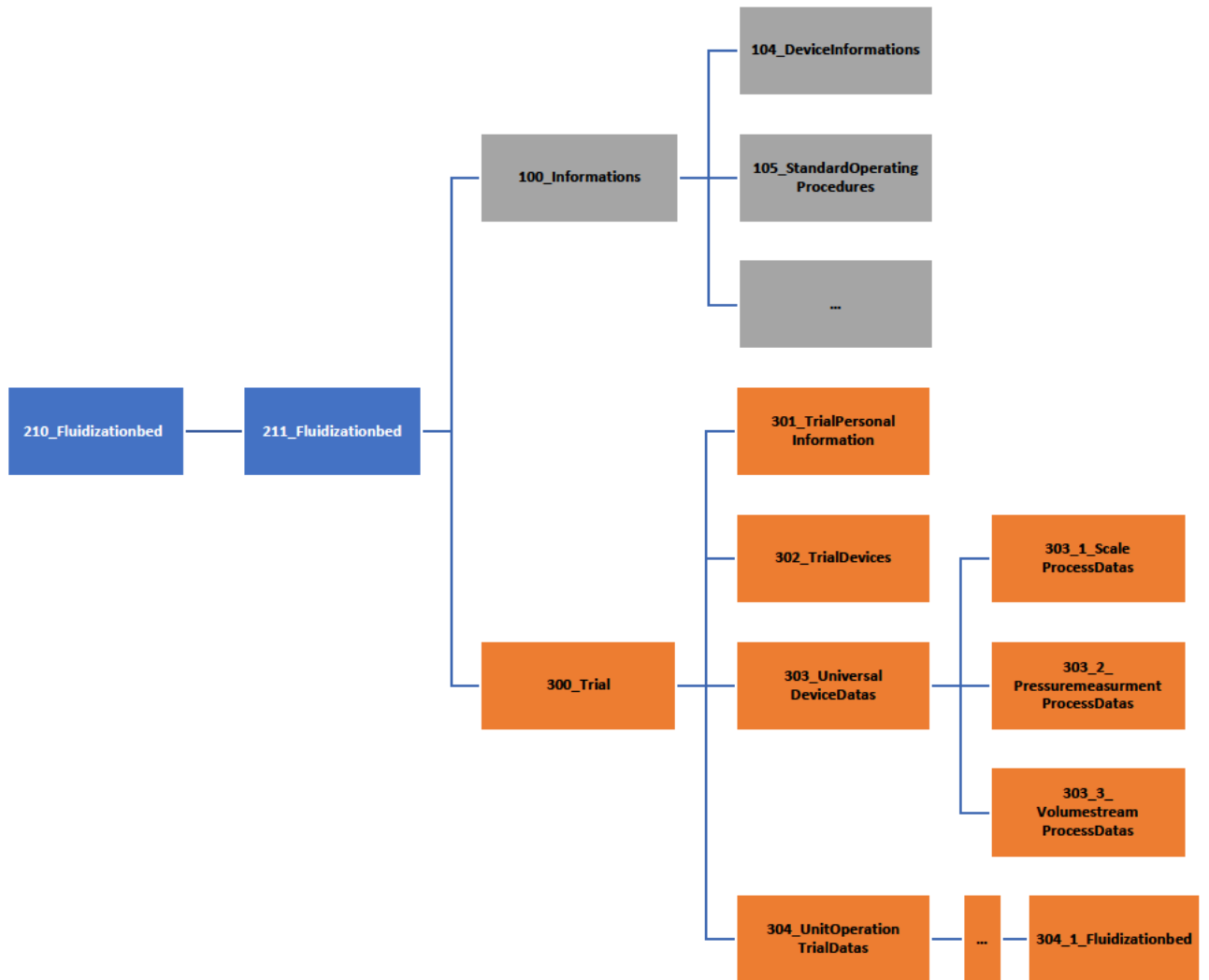
Abbildung 31: Potentielle hierarchische Datenstruktur der Wirbelschicht ( engl. fluidizationbed ) Unit Operation, angelehnt an ISA-S95 und B2MML
