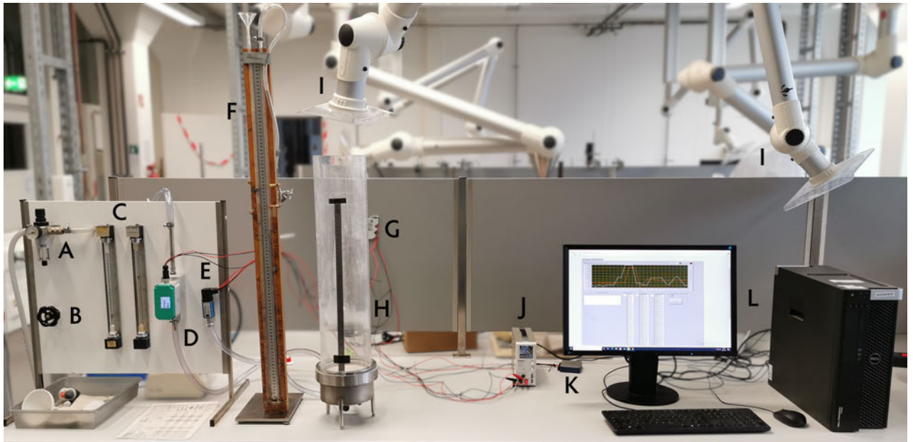
(a) Wirbelschichtversuchsanlage nach den Modifikationen
