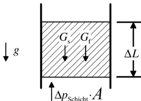
Abbildung 10: Wirbelschichtkräftegleichgewicht an einem Wirbelschichtelement der Länge \Delta L und Anströmfläche A , angelehnt an [41, S. 1562]
