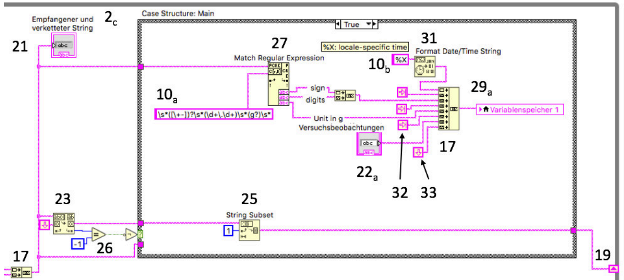
Abbildung 42: String-/Zeilenkonstruktion
