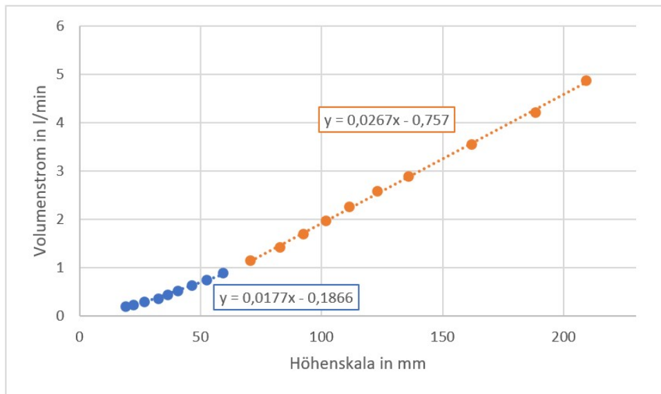
Abbildung 84: Schwebekörperdurchflussmesser ( m=0,6585 g) mit einer Messspanne von 0,185 bis 5 l/min, zzgl. Approximationsfunktionen der Kennlinie
