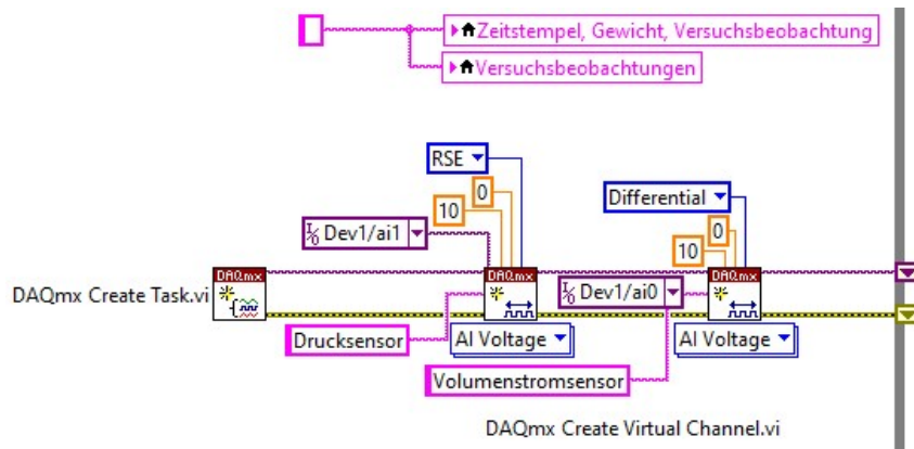
(a) Druck- und Volumenstromsensor Initialisierung der Wirbelschicht
