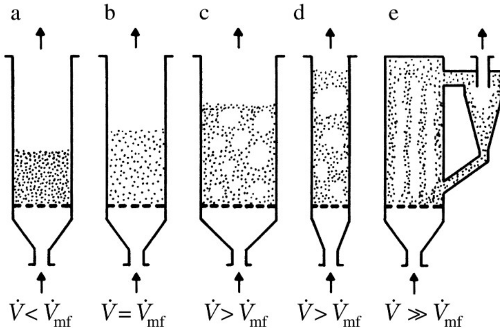
Abbildung 9: Wirbelschichtzustände als Funktion der Anströmgeschwindigkeit [41, S. 1562]
