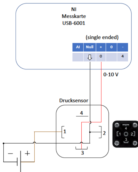
Abbildung 61: Elektrotechnische Verschaltung der Komponenten der Filterkuchenversuchsanlage
