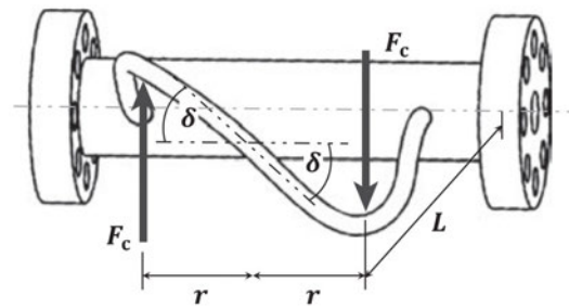
(d) angeregter Coriolissensor mit Durchsatz
