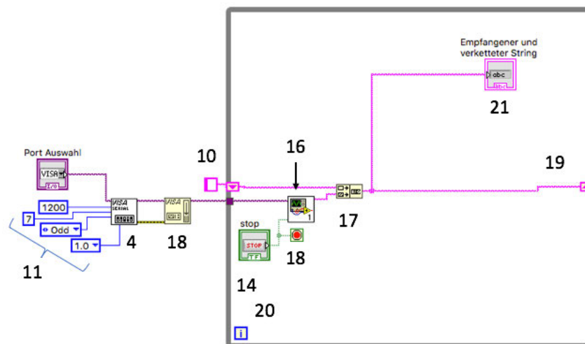
Abbildung 38: BD Haupt VI: SSVI Integration, Port Konfiguration, String auslesen und verketteten
