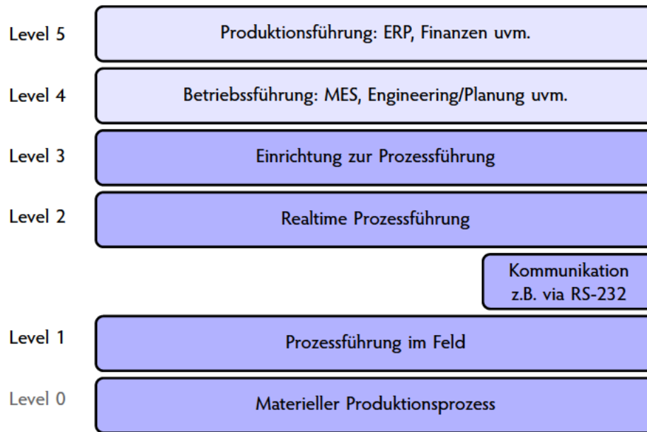
Abbildung 23: ICS-PERA Model, angelehnt an der Grafik des Bundesamtes für Sicherheit in der Informationstechnik des ICS-Kompodiums (vgl. Abbildung 68 im Anhang ; [40, S. 18])
