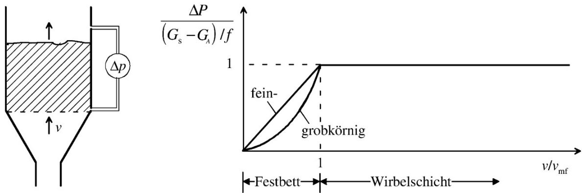
Abbildung 11: Konstanz des dimensionslosen Drucks, ab dem überschreiten der Lockerungsgeschwindigkeit v_{mf} in Anlehnung an [41, S. 1563]
