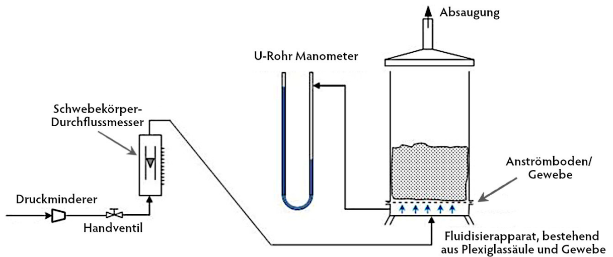
(b) Schematische Skizze des Wirbelschichtversuchs vor den Modifikationen
