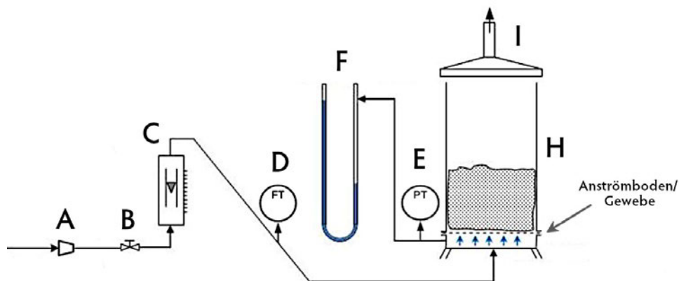
(b) Fließschema in Form einer schematischen Skizze der Wirbelschichtversuchsanlage nach den Modifikationen
