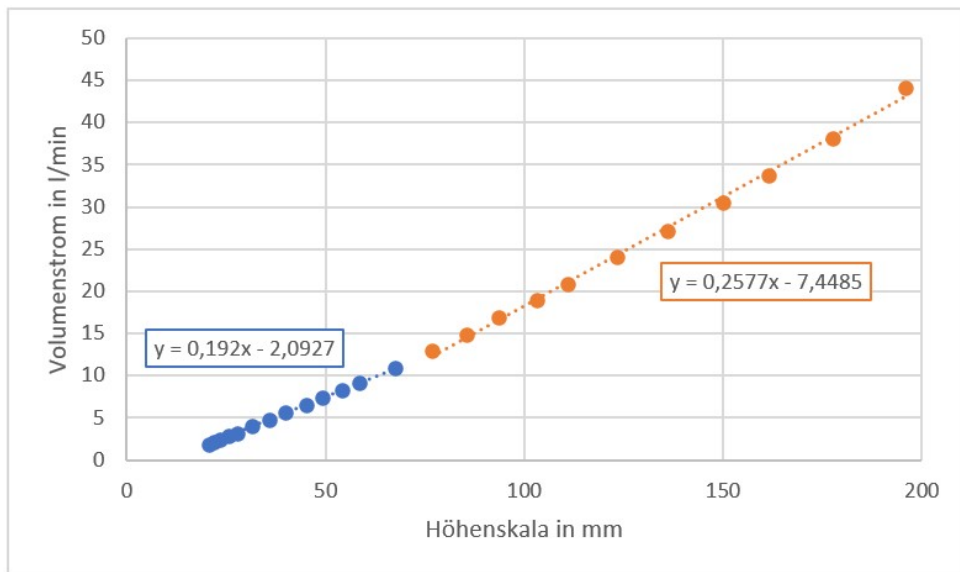
Abbildung 85: Schwebekörperdurchflussmesser ( m=2,225 g) mit einer Messspanne von 1,86 l/min bis 50 l/min, zzgl. Approximationsfunktionen der Kennlinie
