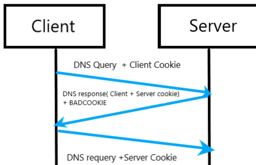
Abbildung 3.8: DNS-Verbindung via DNS Cookies: Entwurf basierend auf [1].
