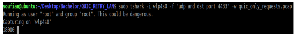
Abbildung 4.6: Paketaufzeichnung der Quiche-Anfragen mit Tshark
