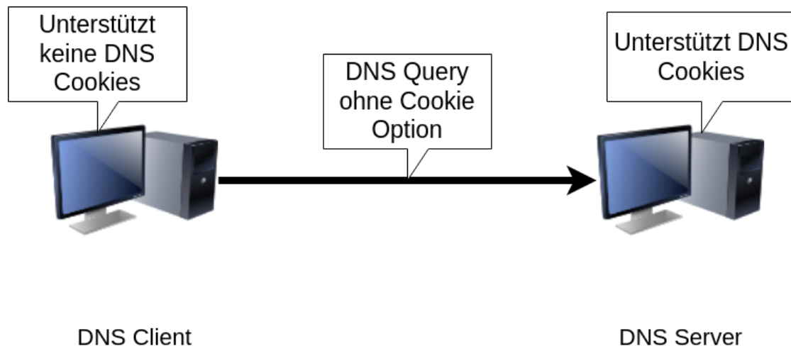
Abbildung 3.6: Client Query ohne Cookie Support. Entwurf basierend auf [1].
