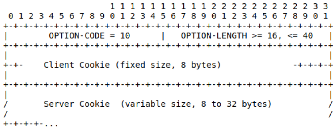
Abbildung 3.7: OPT RR COOKIE OPTION [1].
