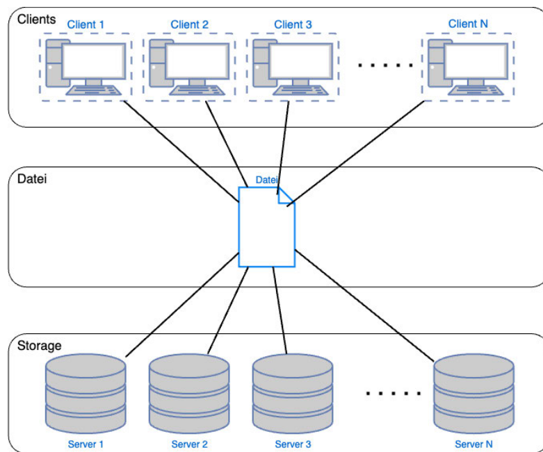
Abbildung 2.3: Paralleler Zugriff mehrerer Clients auf eine Datei, die auf mehreren Speichergeräten verteilt abgelegt ist
