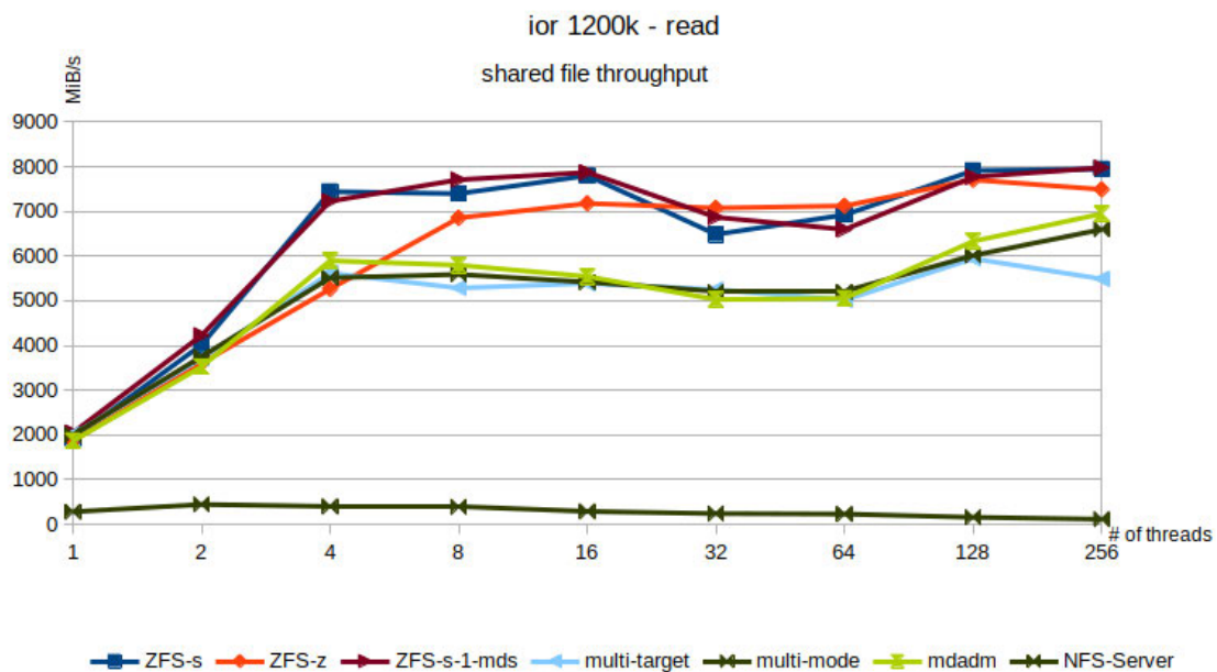
Abbildung 4.3: Shared file throughput (1,2 MB) – Lesevorgang (Abb. ohne ZFS-s-ext4 und ZFS-z-ext4 - vergleichbar mit ZFS-s und ZFS-z )
