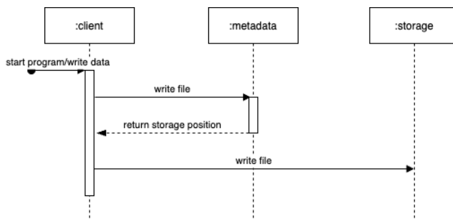
Abbildung 2.6: Schreiben einer neuen Datei/Bearbeiten einer Datei Quelle: Eigene Darstellung
