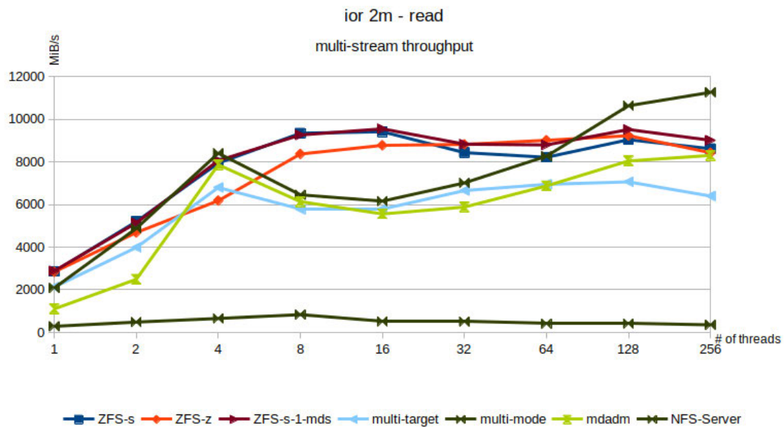
Abbildung 4.1: Multi-stream throughput (2 MiB) – Lesevorgang (Abb. ohne ZFS-s-ext4 und ZFS-z-ext4 - vergleichbar mit ZFS-s und ZFS-z )
