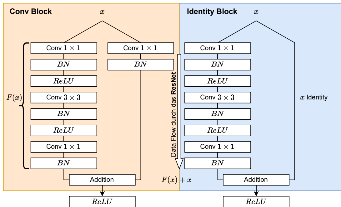
Abbildung 2.3: Residualblöcke: detaillierte Operation innerhalb der Conv - und Identity -Blöcke
