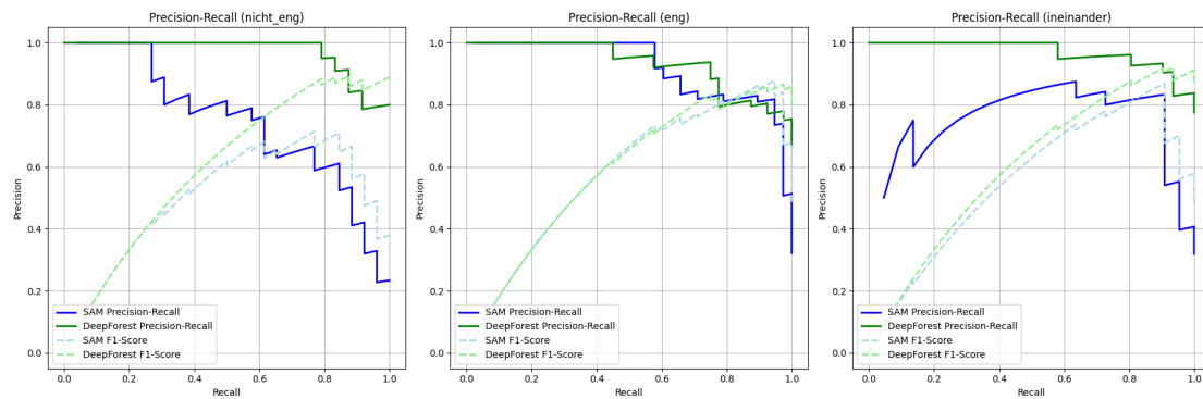
Abbildung 4.11: Precision-Recall-Kurve für San Francisco in den Schwierigkeitsgraden nicht_eng, eng und ineinander
