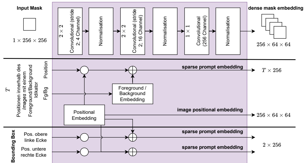
Abbildung 2.9: Detaillierte Darstellung der Funktionsweise des Prompt Encoder in SAM
