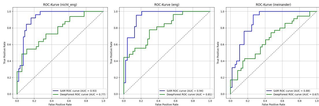
Abbildung 4.8: ROC-Kurve für Kapstadt in den Schwierigkeitsgraden nicht_eng , eng und ineinander
