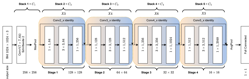
Abbildung 2.4: Detailliertere Darstellung eines ResNet50
