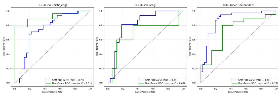
Abbildung 4.16: ROC-Kurve für Tokio in den Schwierigkeitsgraden nicht_eng, eng und ineinander
