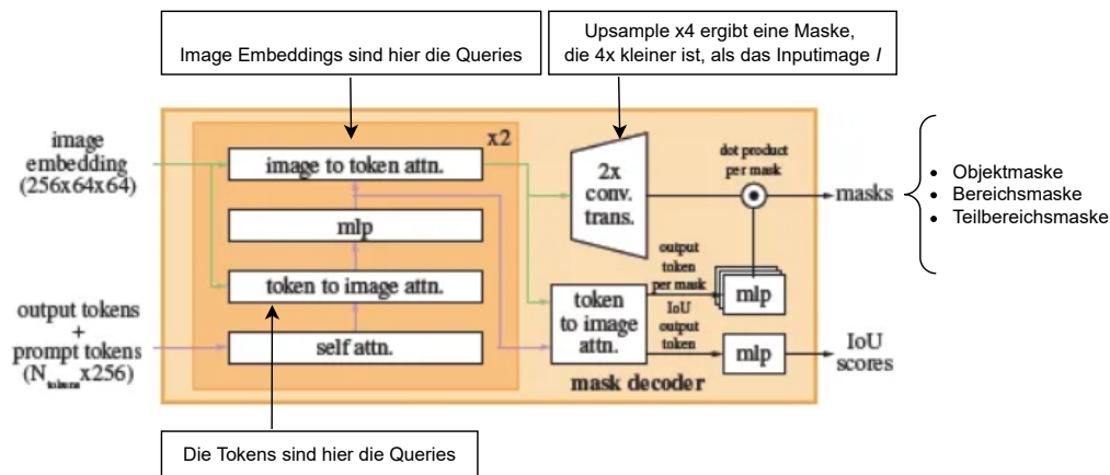
Abbildung 2.10: Schematische Darstellung des Mask Decoders in SAM (angelehnt an[27])
