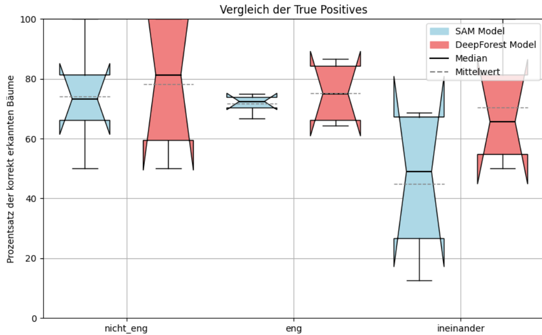
Abbildung 4.9: Boxplot der True Positive Percentage (TP%) für San Francisco in den Schwierigkeitsgraden nicht_eng, eng und ineinander
