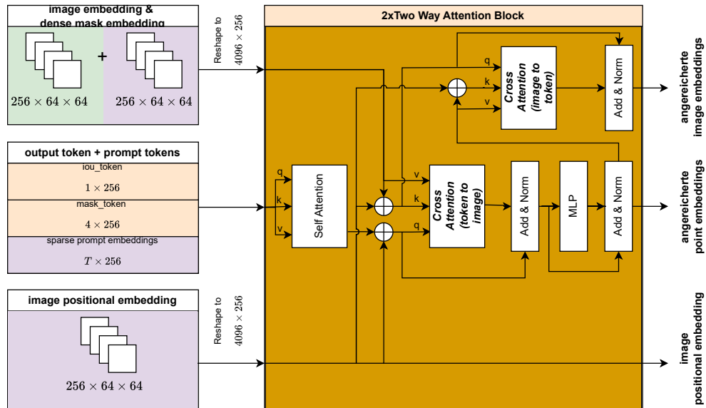
Abbildung 2.11: Eingabeparameter und erste Verarbeitungsschicht des Mask Decoders in SAM
