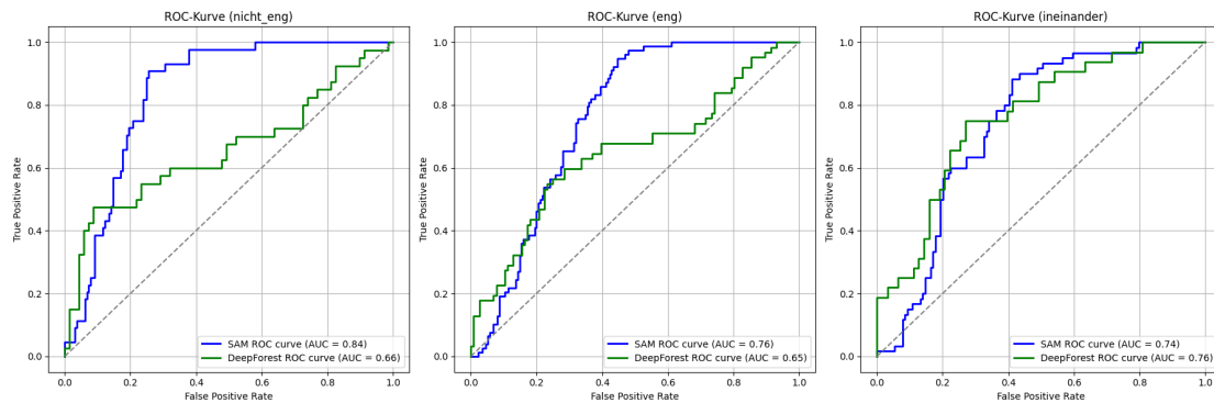
Abbildung 4.4: ROC-Kurve für Hamburg in den Schwierigkeitsgraden nicht_eng , eng und ineinander
