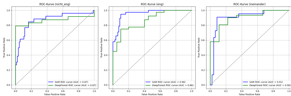
Abbildung 4.12: ROC-Kurve für San Francisco in den Schwierigkeitsgraden nicht_eng , eng und ineinander
