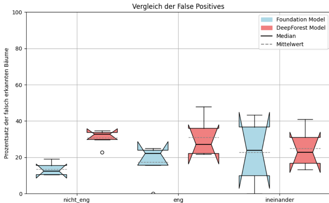
Abbildung 4.6: Boxplot der False Positive Percentage (FP%) für Kapstadt in den Schwierigkeitsgraden nicht_eng, eng und ineinander
