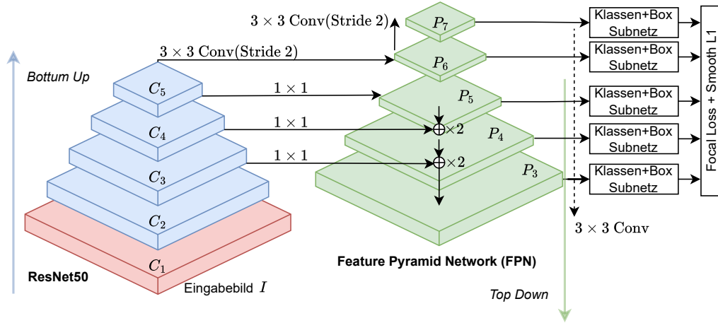
Abbildung 2.5: Die schematische Darstellung eines Feature Pyramid Network (FPN) in grün[31]
