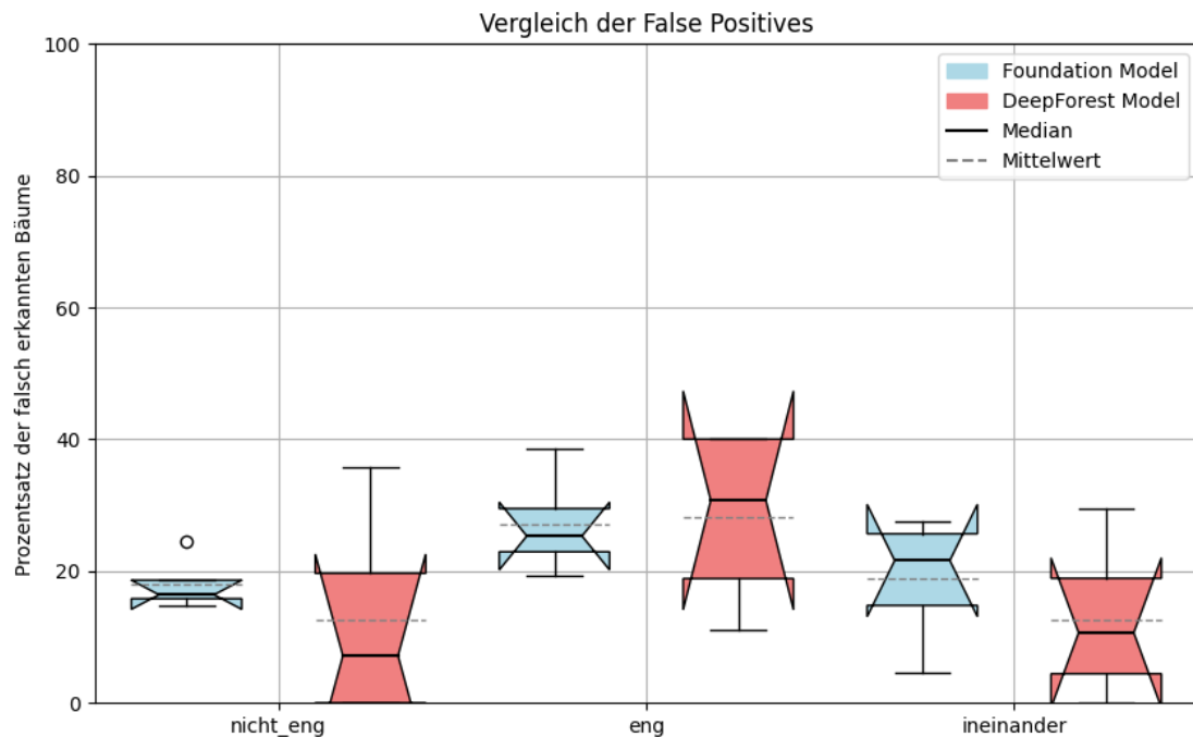
Abbildung 4.10: Boxplot der False Positive Percentage (FP%) für San Francisco in den Schwierigkeitsgraden nicht_eng, eng und ineinander
