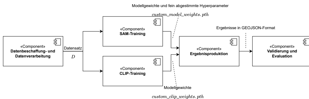
Abbildung 3.1: Komponentendiagramm der implementierten Architektur zur Beantwortung der aufgestellten Hypothesen.
