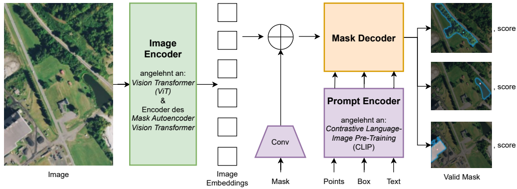
Abbildung 2.6: Segment Anything Model (SAM) Architekturübersicht (angelehnt an[27])
