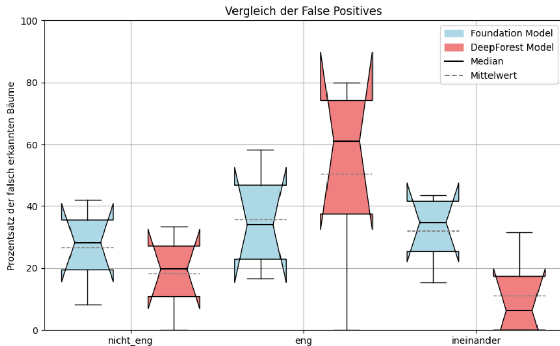
Abbildung 4.14: Boxplot der False Positive Percentage (FP%) für Tokio in den Schwierigkeitsgraden nicht_eng, eng und ineinander
