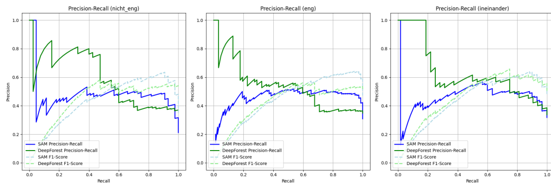
Abbildung 4.3: Precision-Recall-Kurve für Hamburg in den Schwierigkeitsgraden nicht_eng , eng und ineinander
