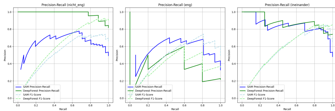
Abbildung 4.15: Precision-Recall-Kurve für Tokio in den Schwierigkeitsgraden nicht_eng, eng und ineinander
