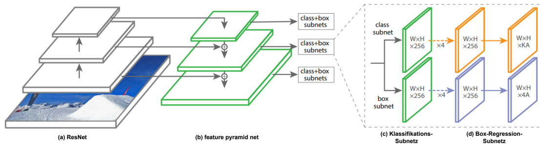
Abbildung 2.1: Die schematische Darstellung eines RetinaNet[32]
