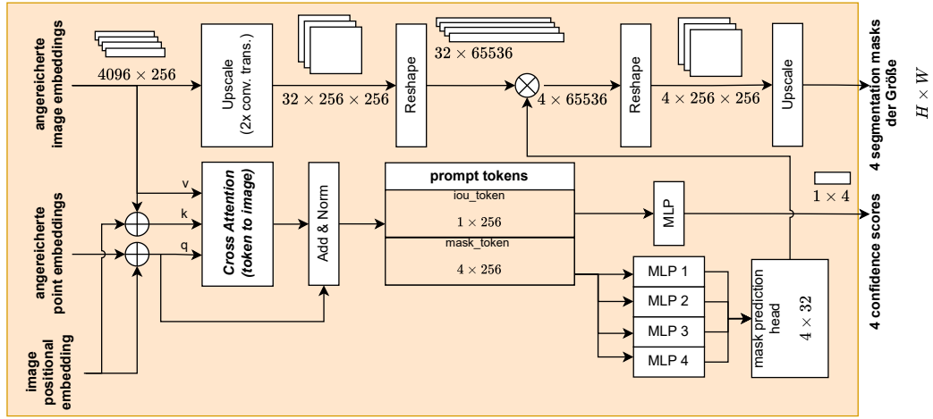
Abbildung 2.12: Eingabeparameter und zweite Verarbeitungsschicht des Mask-Decoders in SAM
