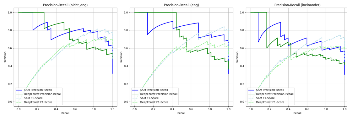
Abbildung 4.7: Precision-Recall-Kurve für Kapstadt in den Schwierigkeitsgraden nicht_eng, eng und ineinander
