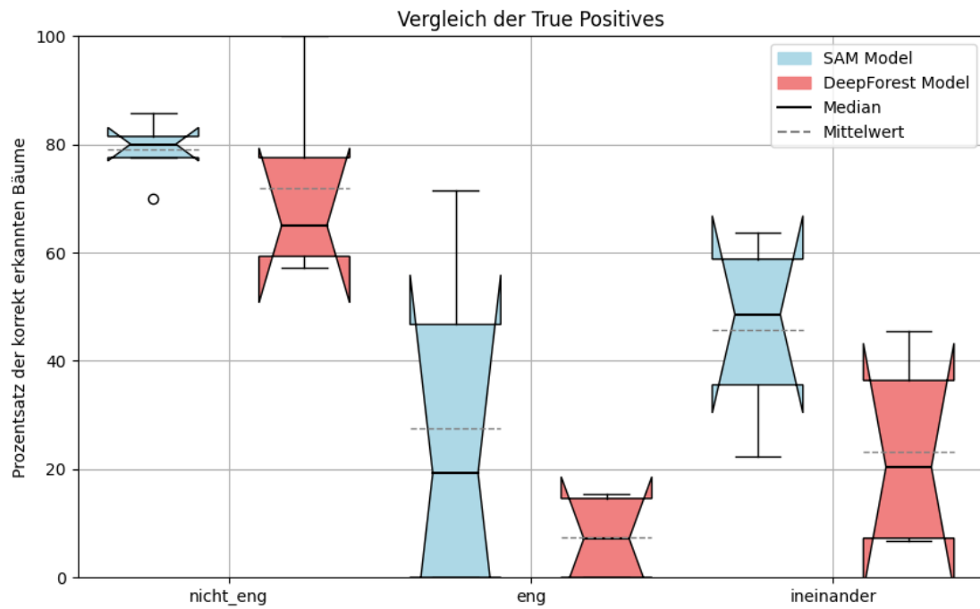
Abbildung 4.13: Boxplot der True Positive Percentage (TP%) für Tokio in den Schwierigkeitsgraden nicht_eng, eng und ineinander
