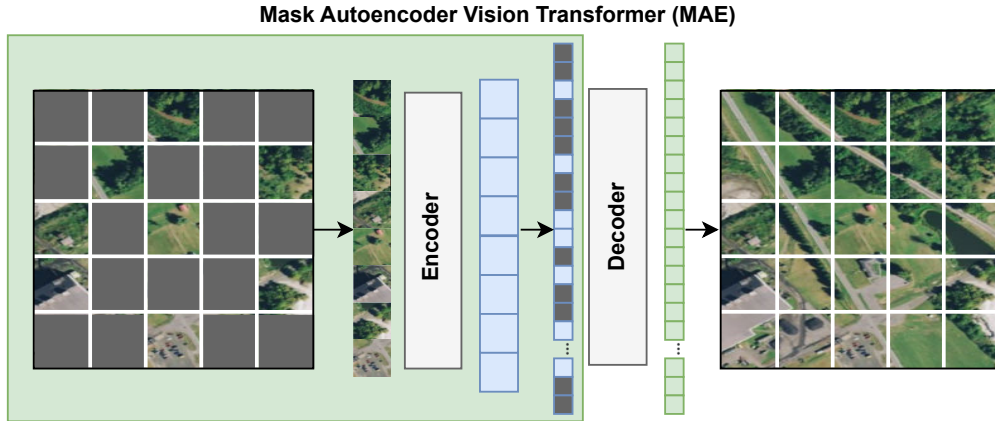
Abbildung 2.8: MAE-Strategie zur Repräsentationsgewinnung im SAM (nur Encoder-Teil)
