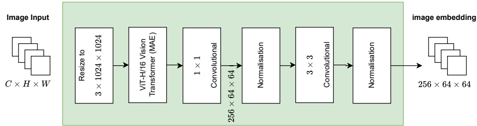
Abbildung 2.7: Der Image Encoder des Segment Anything Model (SAM)
