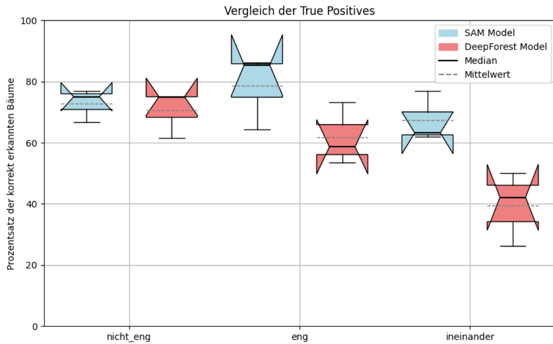
Abbildung 4.1: Boxplot der True Positive Percentage (TP%) für Hamburg in den Schwierigkeitsgraden nicht_eng, eng und ineinander
