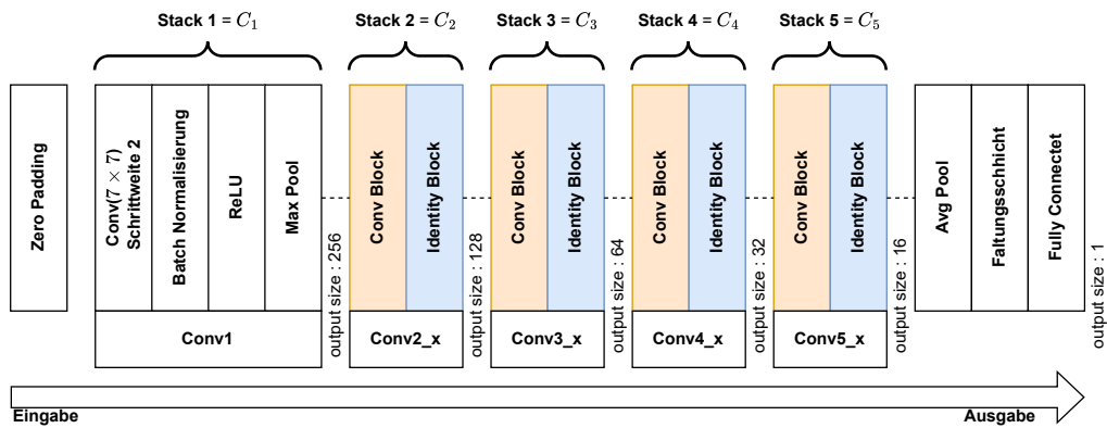
Abbildung 2.2: ResNet Backbone (angelehnt an [18])
