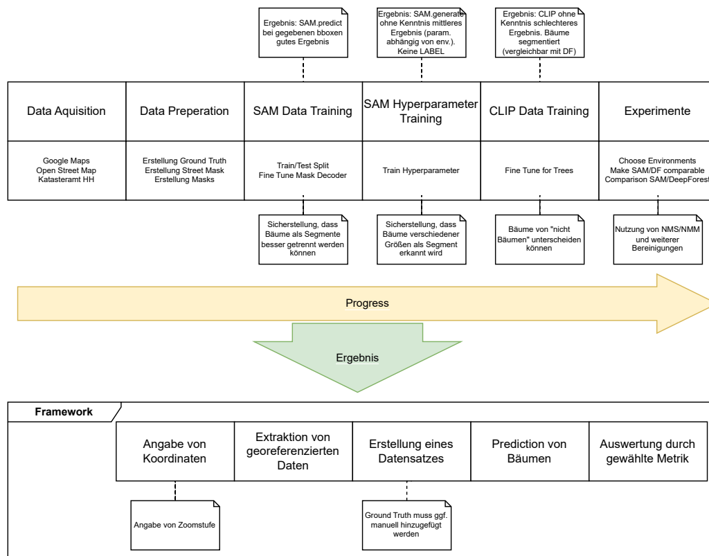
Abbildung 3.6: Überblick des implementierten Frameworks zur Beantwortung der in der Arbeit gestellten Hypothesen.
