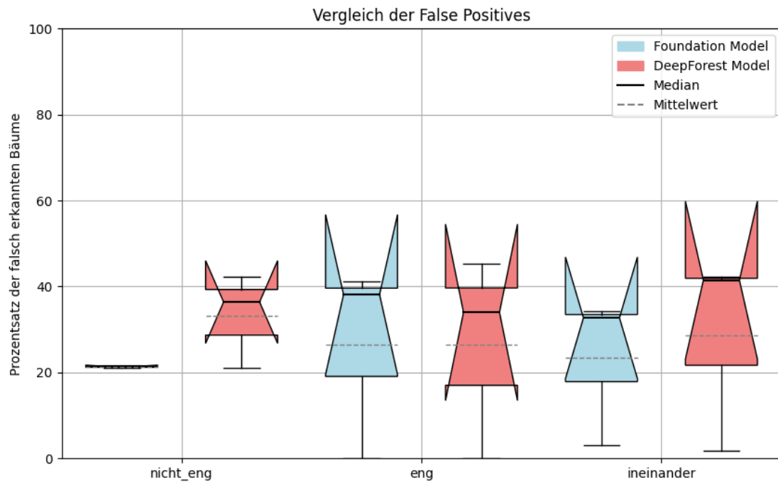
Abbildung 4.2: Boxplot der False Positive Percentage (FP%) für Hamburg in den Schwierigkeitsgraden nicht_eng, eng und ineinander
