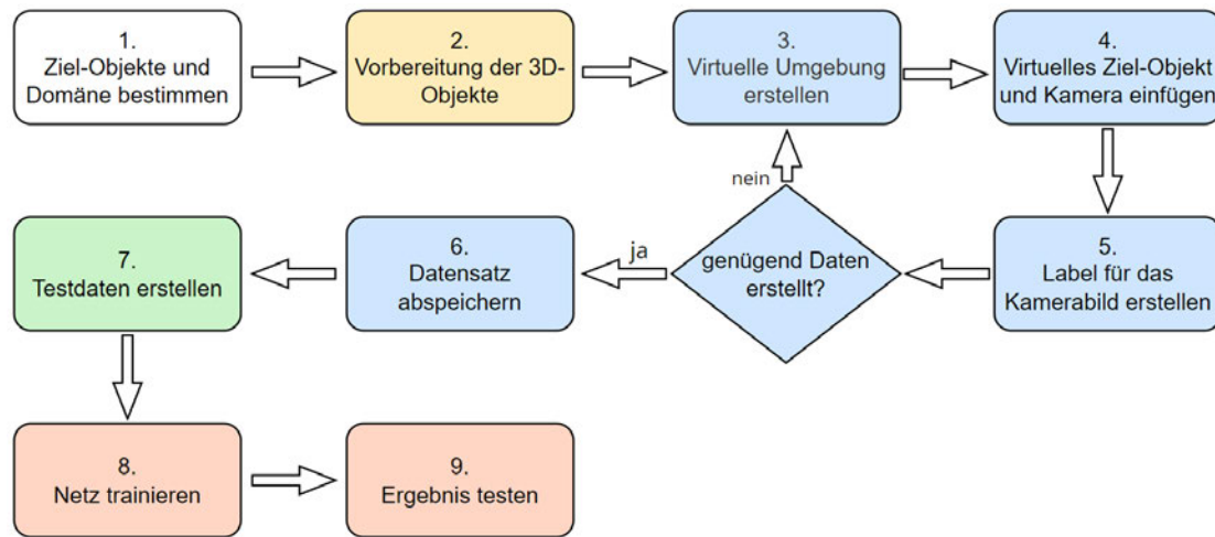
Abbildung 3.3: Ablauf der Experimente, Quelle: Eigene Abbildung
