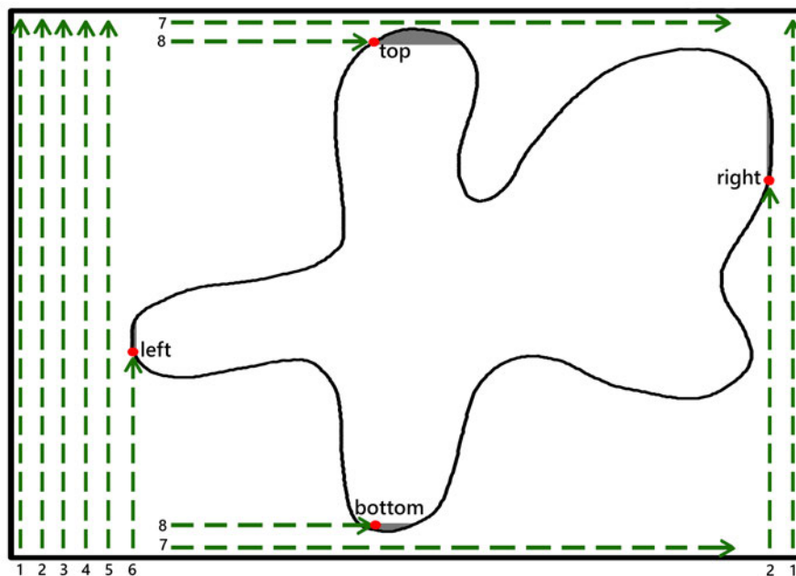
Abbildung 4.5: Algorithmus zur Bestimmung der 2D-Grenzen eines Objekts
