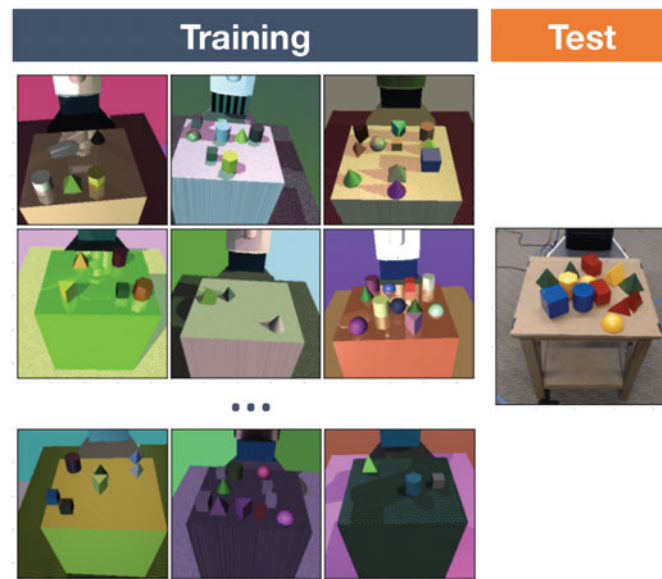
Abbildung 2.7: Auszug aus den generierten Trainingsdaten im Vergleich zu realen Testdaten
