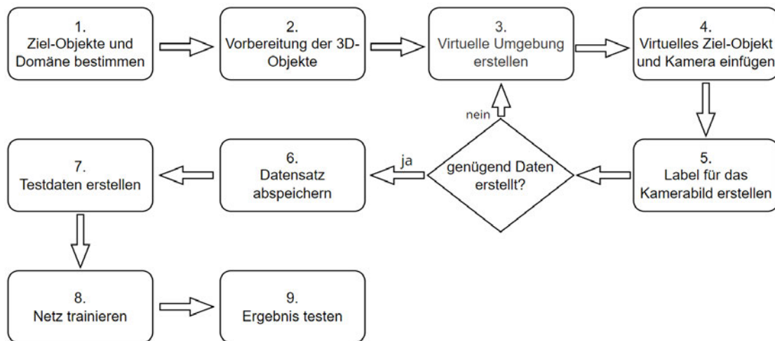
Abbildung 3.1: Ablauf der Experimente, Quelle: Eigene Abbildung
