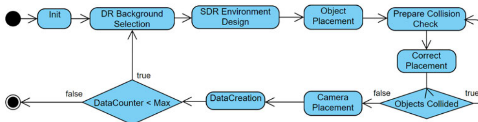
Abbildung 4.2: Zustandsdiagramm der Anwendung, Quelle: Eigene Abbildung
