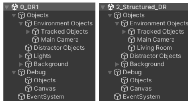
Abbildung 4.3: Hierarchien der Szenen DR1 und SDR1, Quelle: Eigene Abbildung
