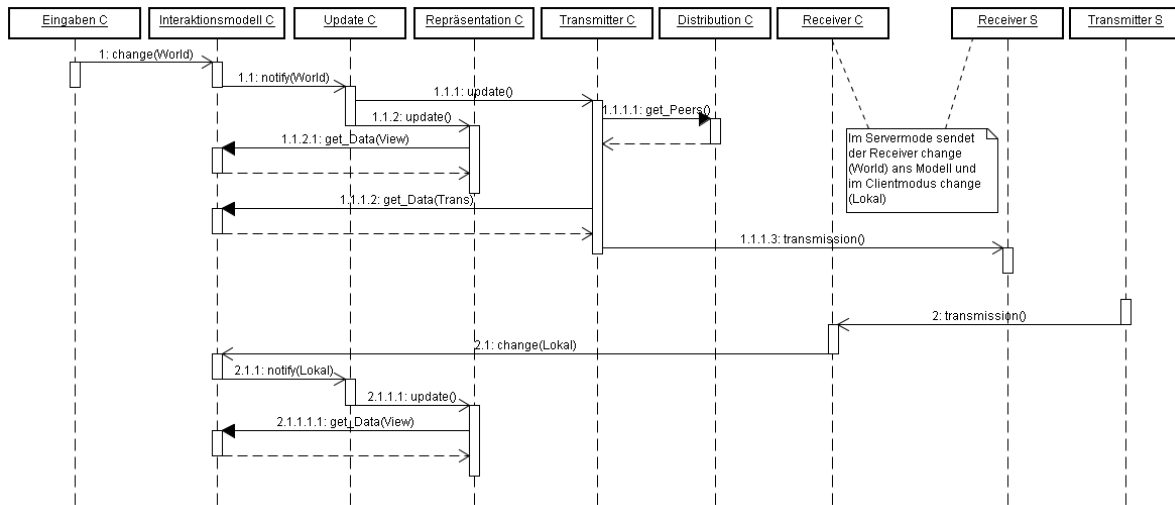
Abbildung 4.25: Clientseitiges Sequenzdiagramm.
