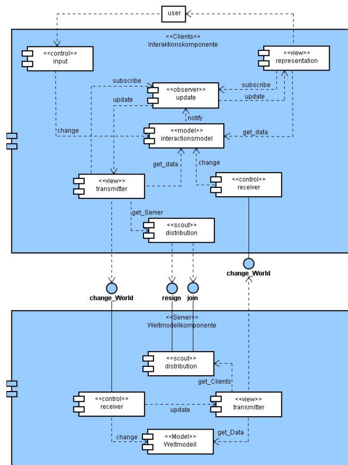
Abbildung 4.16: Entwicklungsschritt der Architektur mit unabhängigem Modell und angelegter Client-Server- Distribution.
