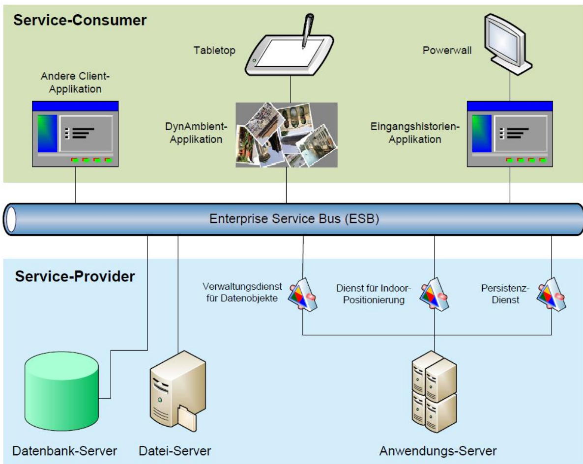
Abbildung 4.32: Vorgeschlagene übergeordnete Architektur für DynAmbient von (Roßberger, 2008).
