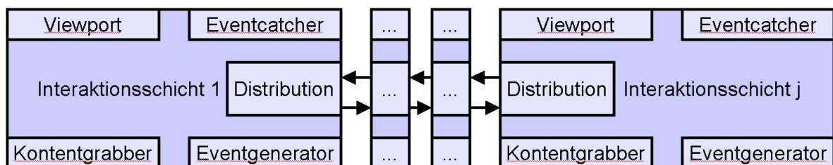
Abbildung 4.4: Der Status der Interaktionsschicht wird durch die Distributionskomponente über das Gesamtsystem verteilt.
