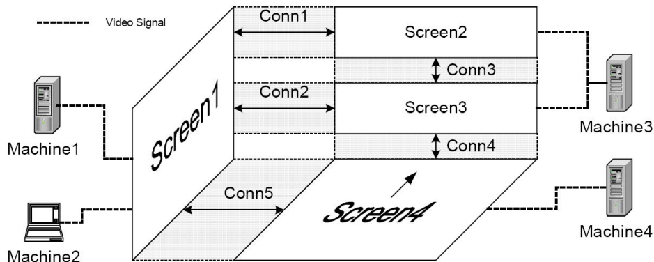
Abbildung 2.7: Screens sind in der virtuellen Topologie ähnlich der realen Welt angeordnet und die Verbindungen zwischen den Bildschirmen für den Übertritt von Mauszeigern sind zwischen den Screens definiert. (Aus (Johanson u. a., 2001))
