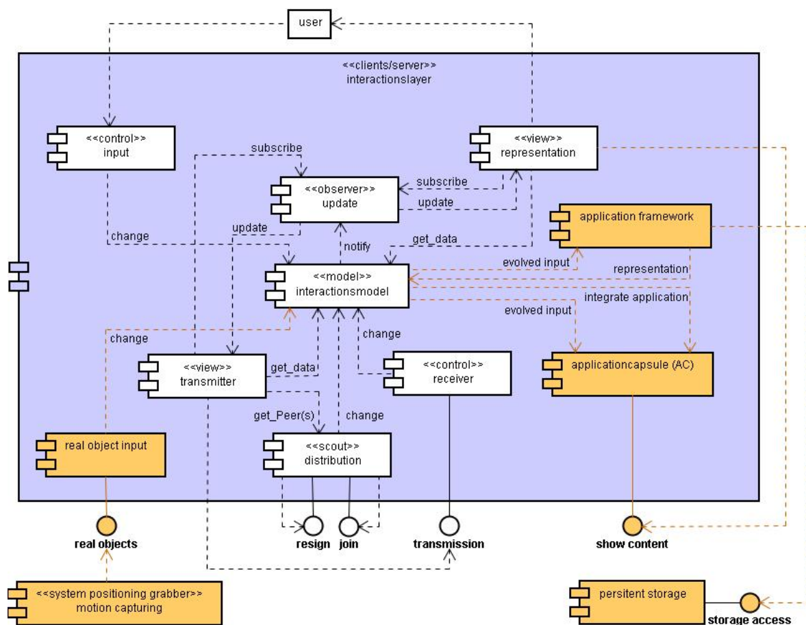
Abbildung 4.28: Die Architektur des Interaktionslayer erweitert durch drei Komponenten.
