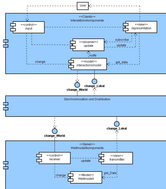
Abbildung 4.15: Systemarchitektur mit Ausgliederung der Distribution und notwendiger Erweiterung durch das Observer-Pattern.
