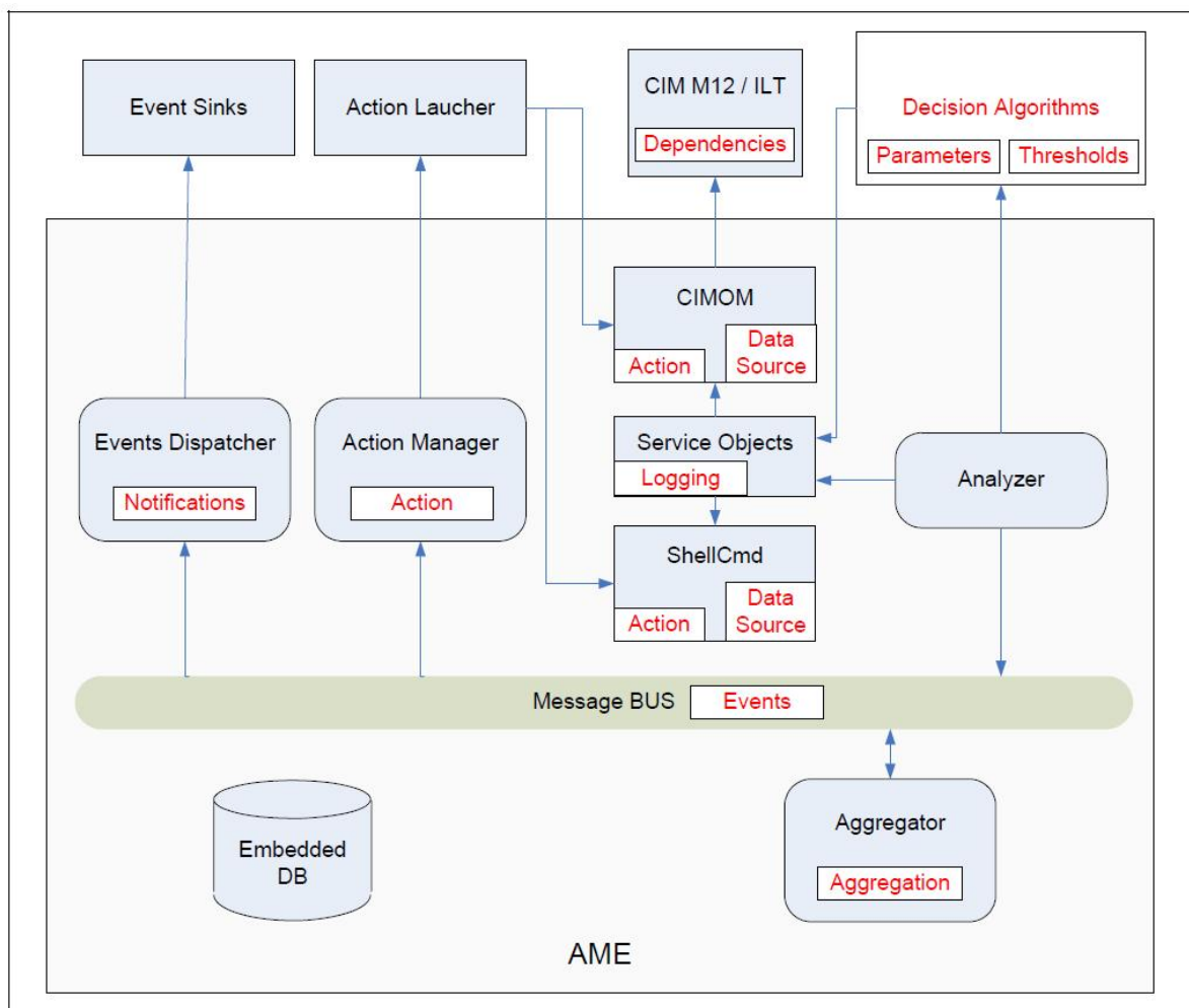
Abbildung 4.31: Die Architektur der Autonomic Management Engine (AME). (Manoel u. a., 2005)
