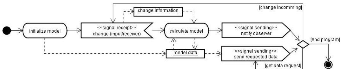
Abbildung 4.21: Interaktionsmodellkomponente.
