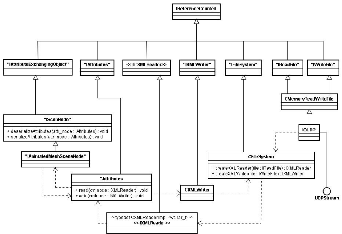
Abbildung 5.7: Die erweiterte Serialisierungsmechanik in Irrlicht.
