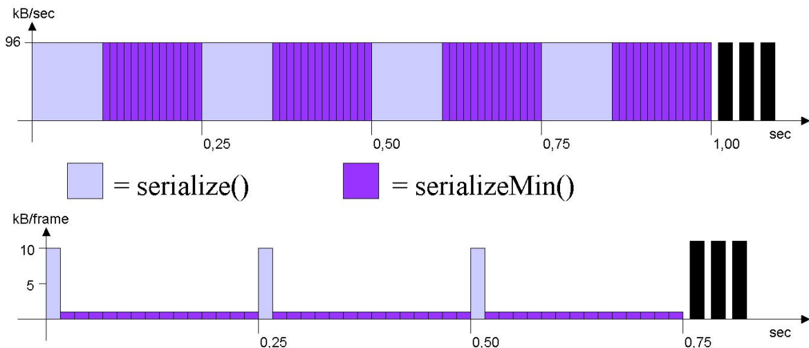
Abbildung 5.6: Die Datenübertragungsrates würde ohne die Komprimierung in diesem Beispiel das sechsfache betragen und die mögliche Framerate bei beschränkter Kanalkapazität ein sechstel.
