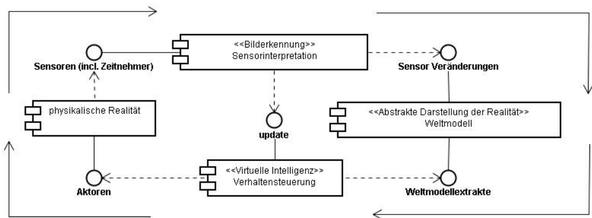
Abbildung 4.8: Verallgemeinerte Darstellung einer Architektur für Roboterprogrammierung.
