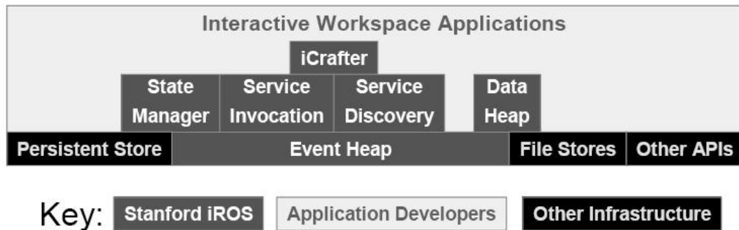
Abbildung 2.6: Struktur der iROS Komponenten. (Aus (Johanson, 2003))
