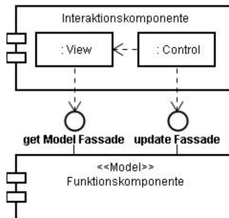
Abbildung 4.12: Einbettung des MVC-Pattern in die Vorgabe zur Evaluierbarkeit.
