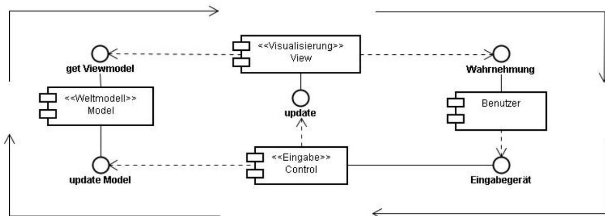
Abbildung 4.9: Allgemeine Darstellung eines Eingabe-Verarbeitung-Ausgabe Systems basierend auf dem MVC-Pattern.
