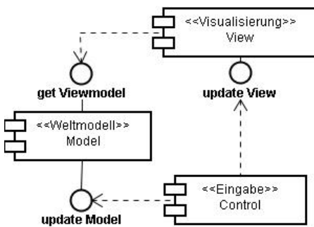
Abbildung 4.10: Das MVC-Pattern.
