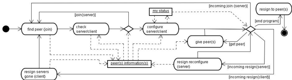
Abbildung 4.24: Distributionskomponente.
