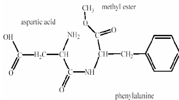
Abb. 1: Strukturformel von Aspartam
