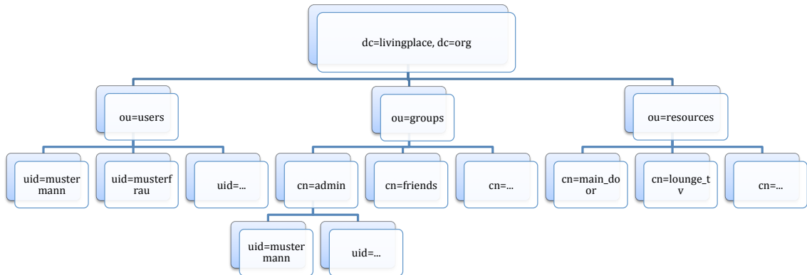
Abbildung 4.1.: LDAP Baumstruktur
