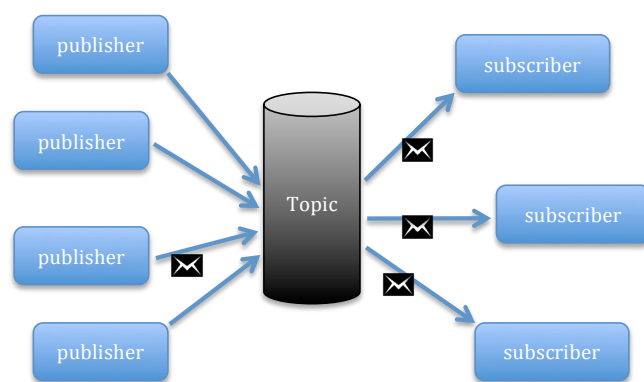
Abbildung 3.1.: Publish-Subscribe Pattern
