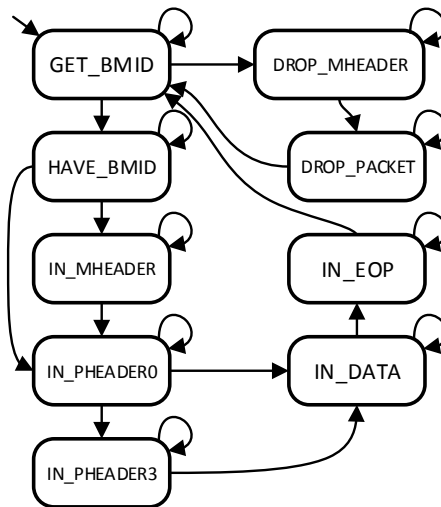
Abbildung 4.13: Mealy-Zustandsautomat der Buffer Sink
