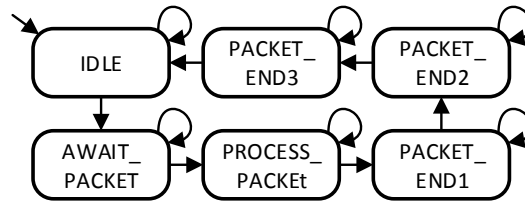
Abbildung 4.17: In CTRL Exec verwendeter Zustandsautomat
