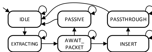
Abbildung 4.15: Mealy-Zustandsautomat des VLAN Taggers
